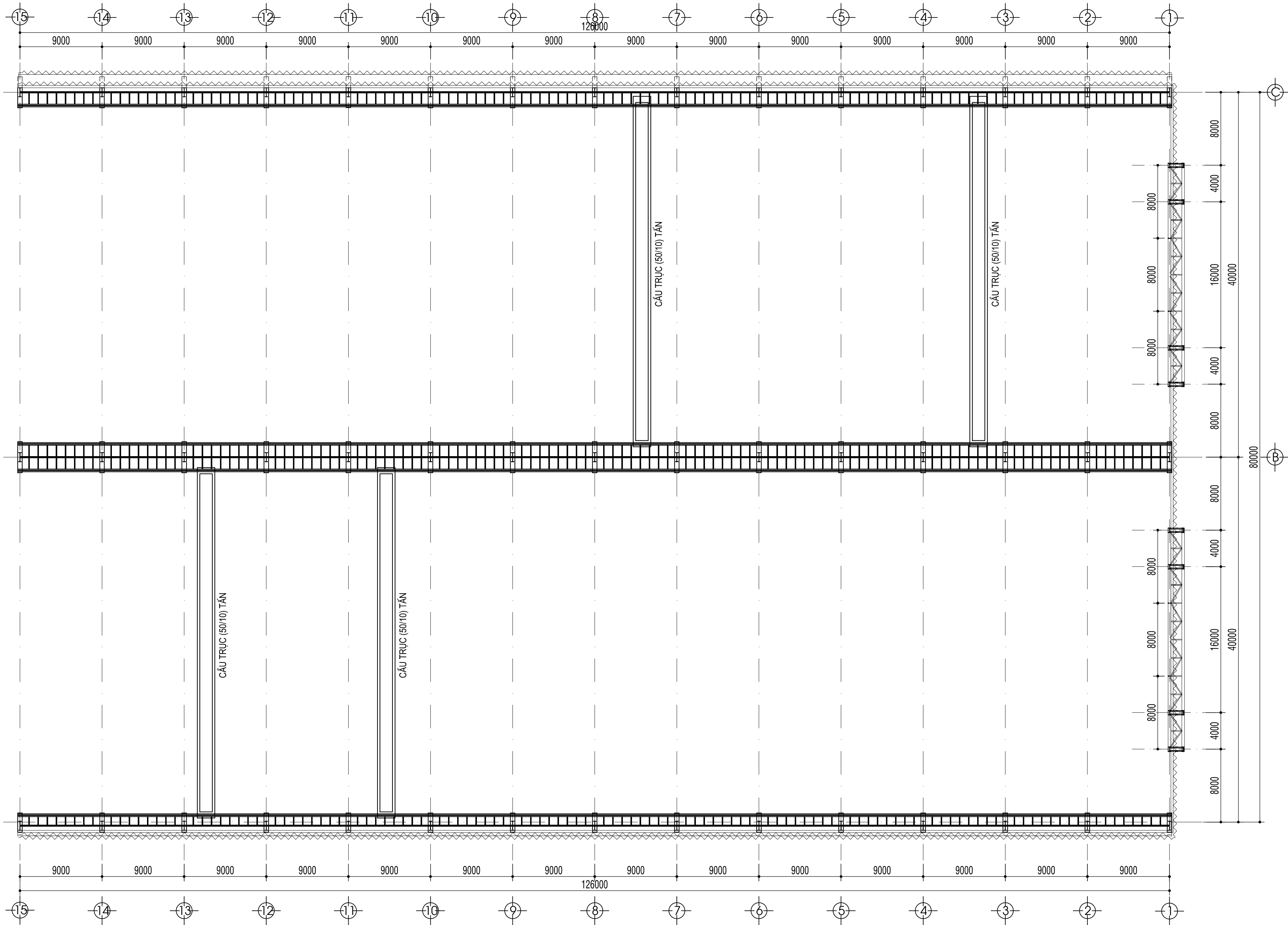
MẶT BẰNG COTE + 18.000 - TL1/200
