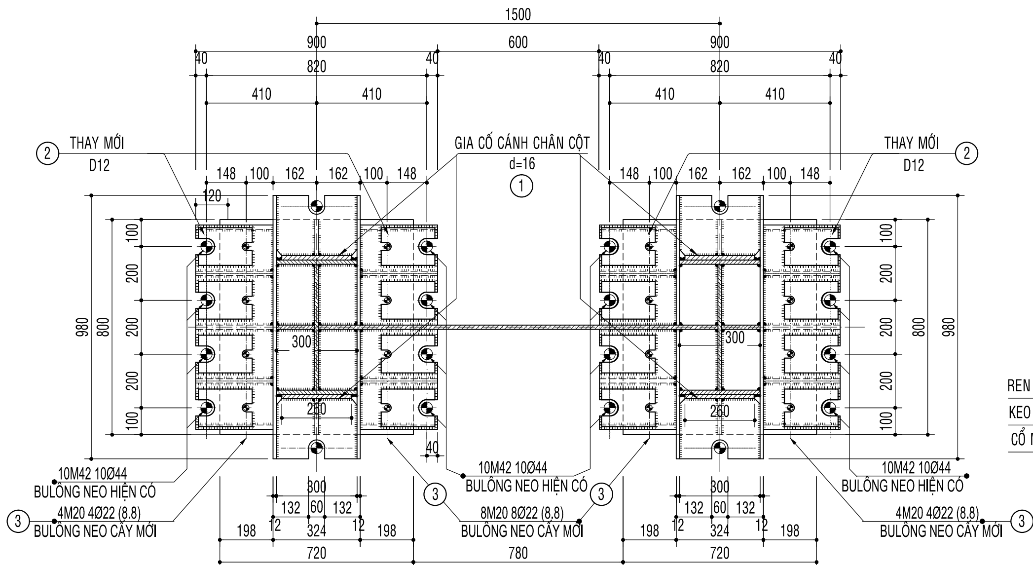
CẮT 1-1
