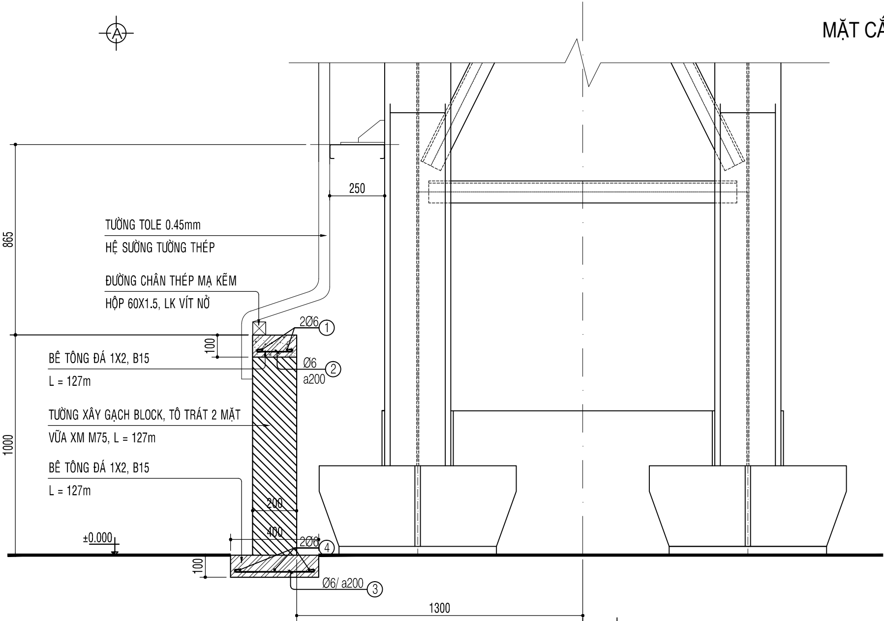
CHÂN TƯỜNG TRỤC A, C
