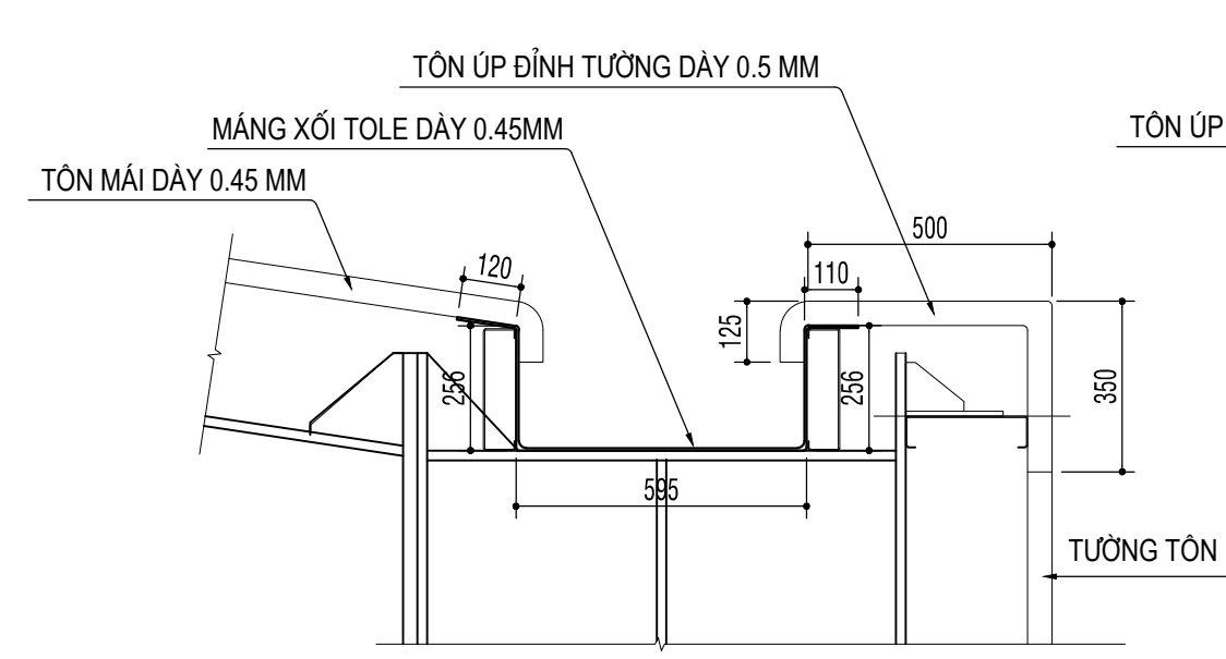
MĂNG XỐI TRỤC C (L=127M)
