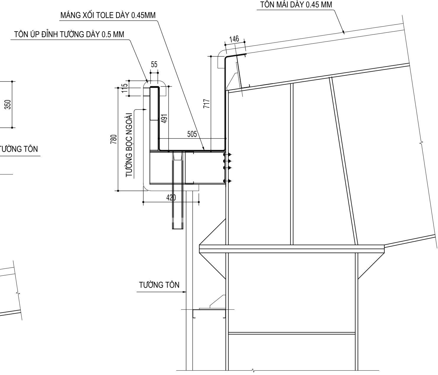
MĂNG XỐI TRỤC A (L=127M)
