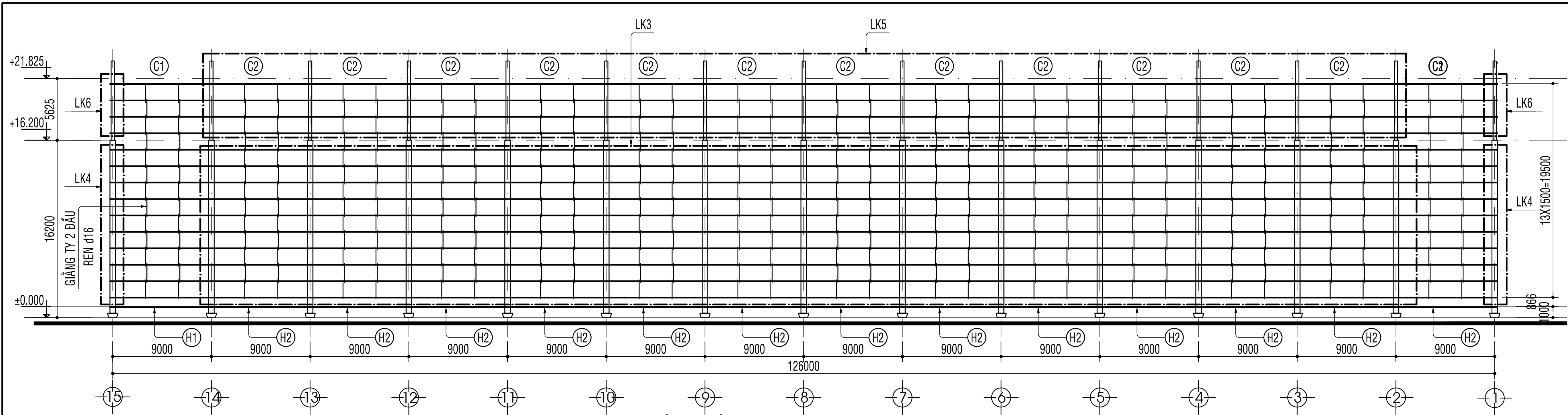
SƯỜN TƯỜNG TRỤC A - TL 1/200
