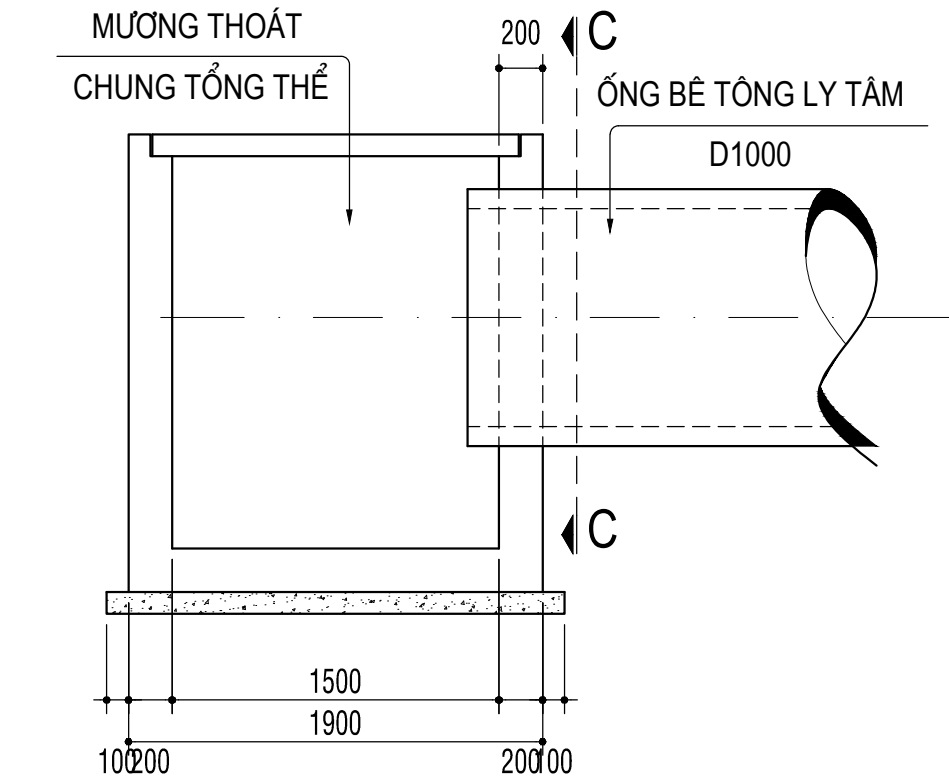
ĐẤU NỐI HỆ THỐNG TỔNG THỂ
