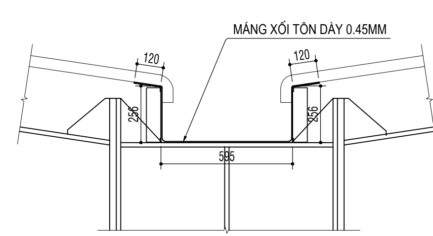
MĂNG XỐI TRỤC B (L=127M)
