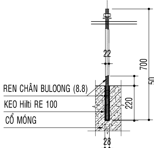
CHI TIẾT KHOAN CẮY BULOÔNG
