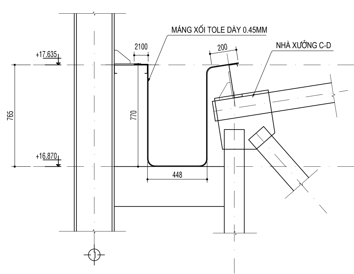
MĂNG XỐI TRỤC 1 (L=82.6M)
