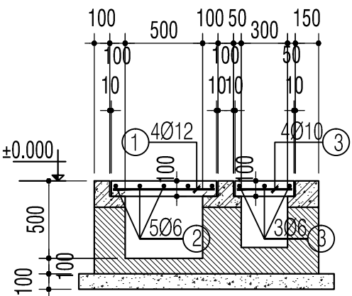
CẮT A-A
