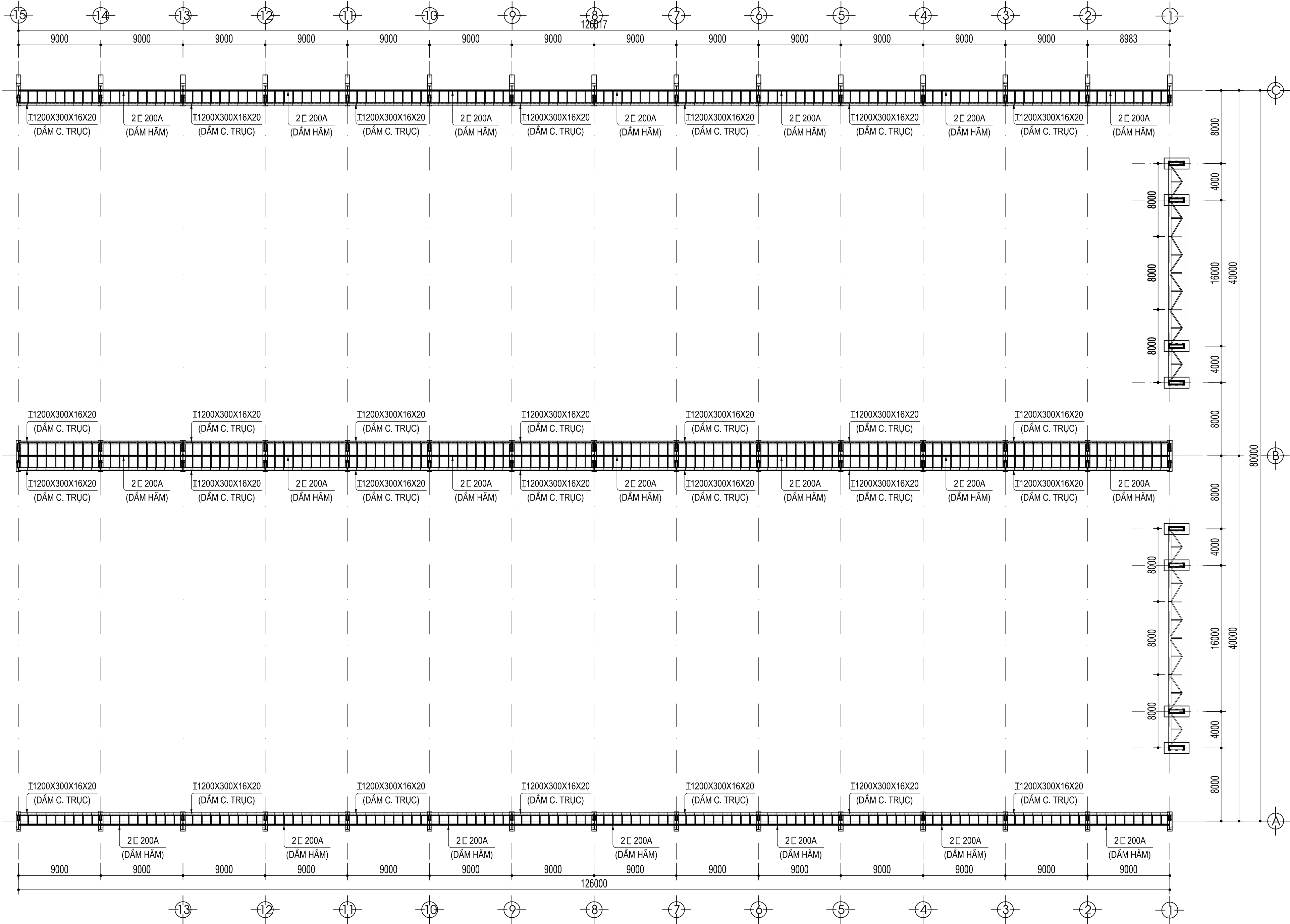
SƠ ĐỒ CẢI TẠO DẦM ĐỖ CẦU TRỤC , THAY MỚI DẦM HẪM
