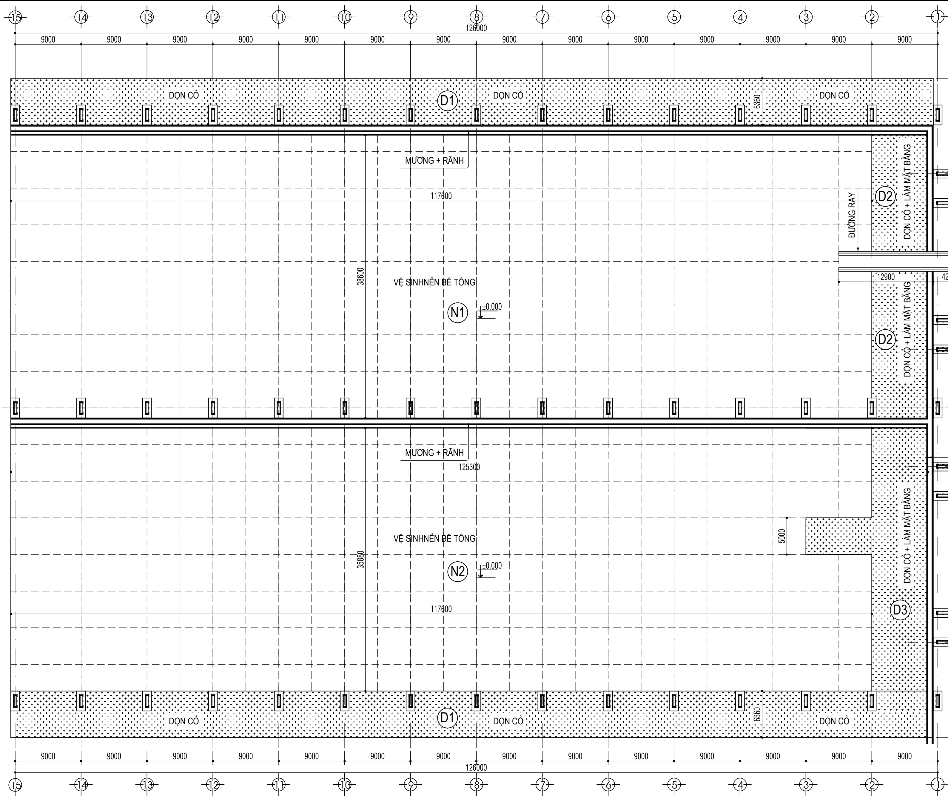
DƠN VỆ SINH MẶT BẰNG - TL1/200
