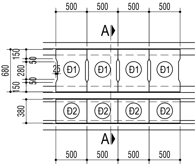
TRÍCH ĐOẠN ĐAN MƯƠNG
