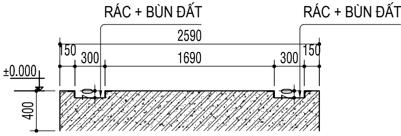
ĐƯỜNG RAY (L=1 X 17.15M)
