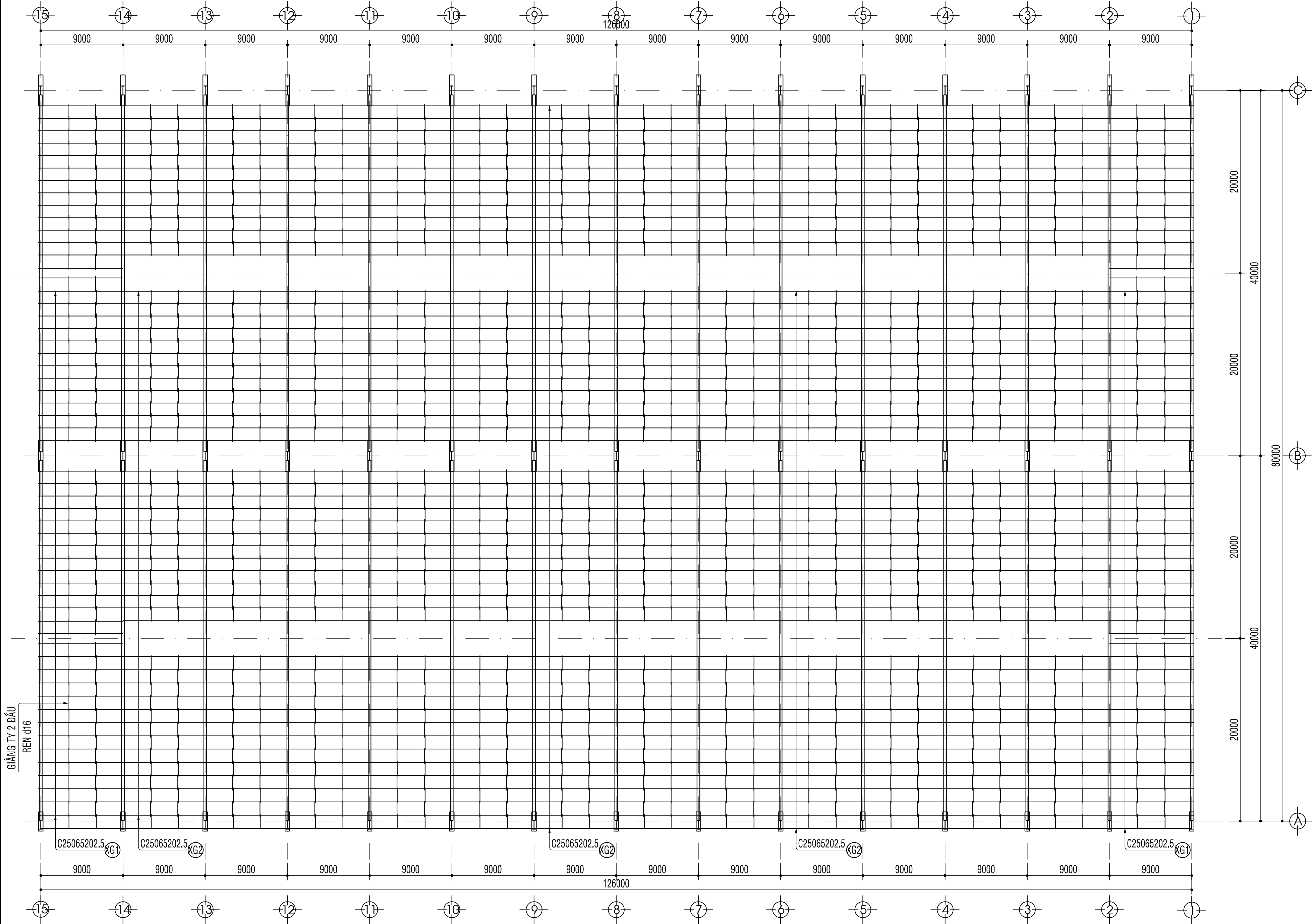
MẶT BẰNG XÀ GỖ MÁI
