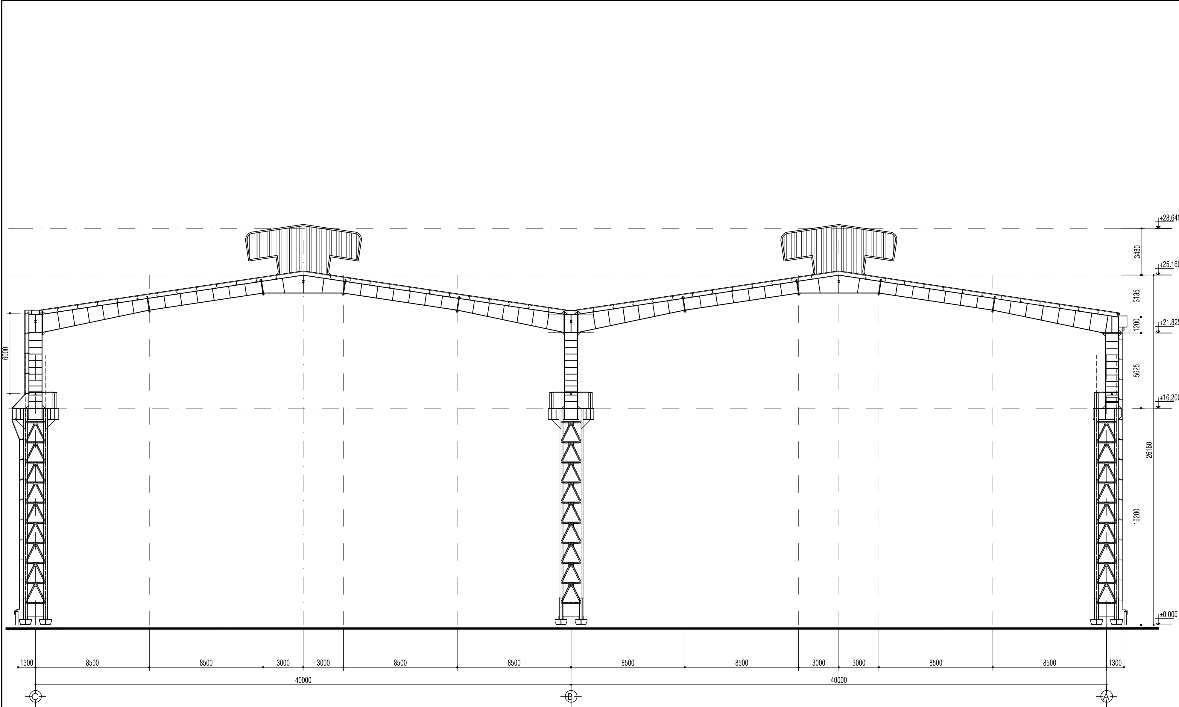
MẶT ĐỨNG TRỤC C - A - TL1/100
