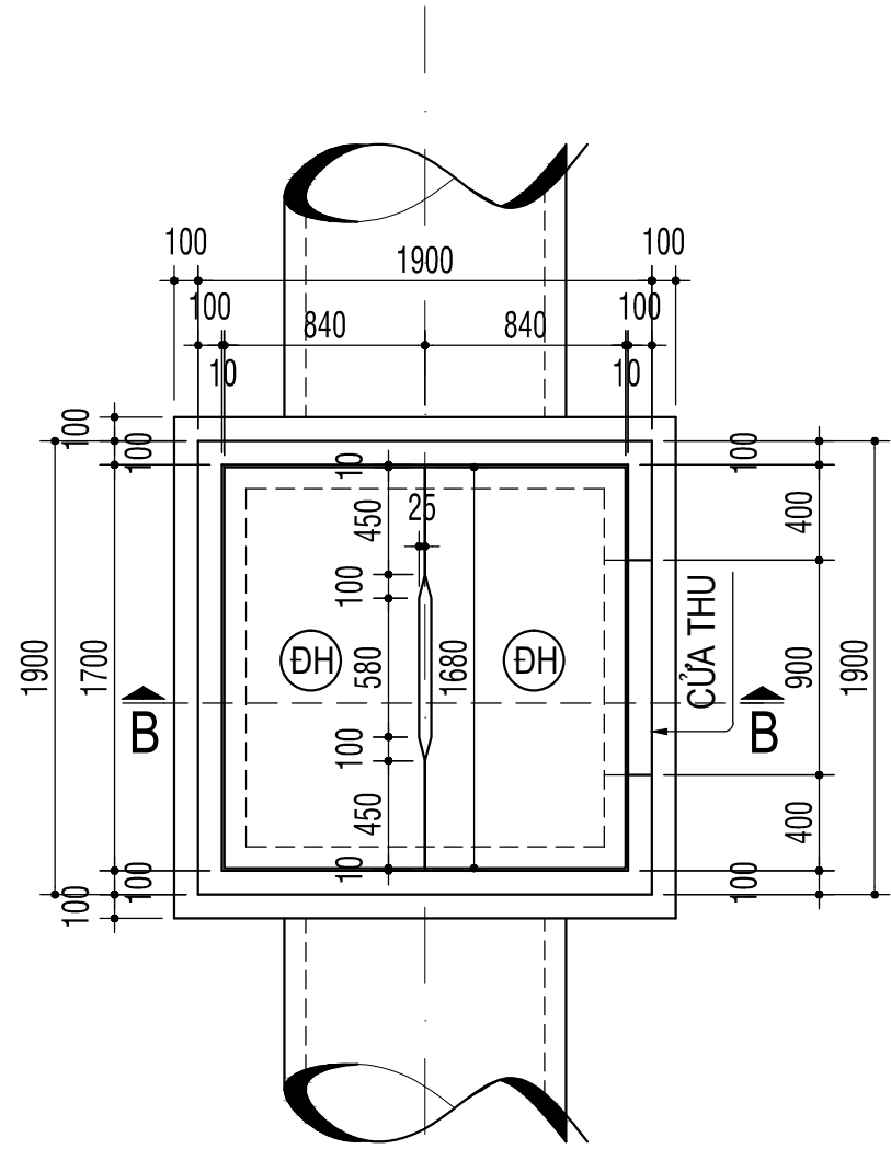
TRÍCH ĐOẠN ỐNG + HỐ GA TRỤC 15
