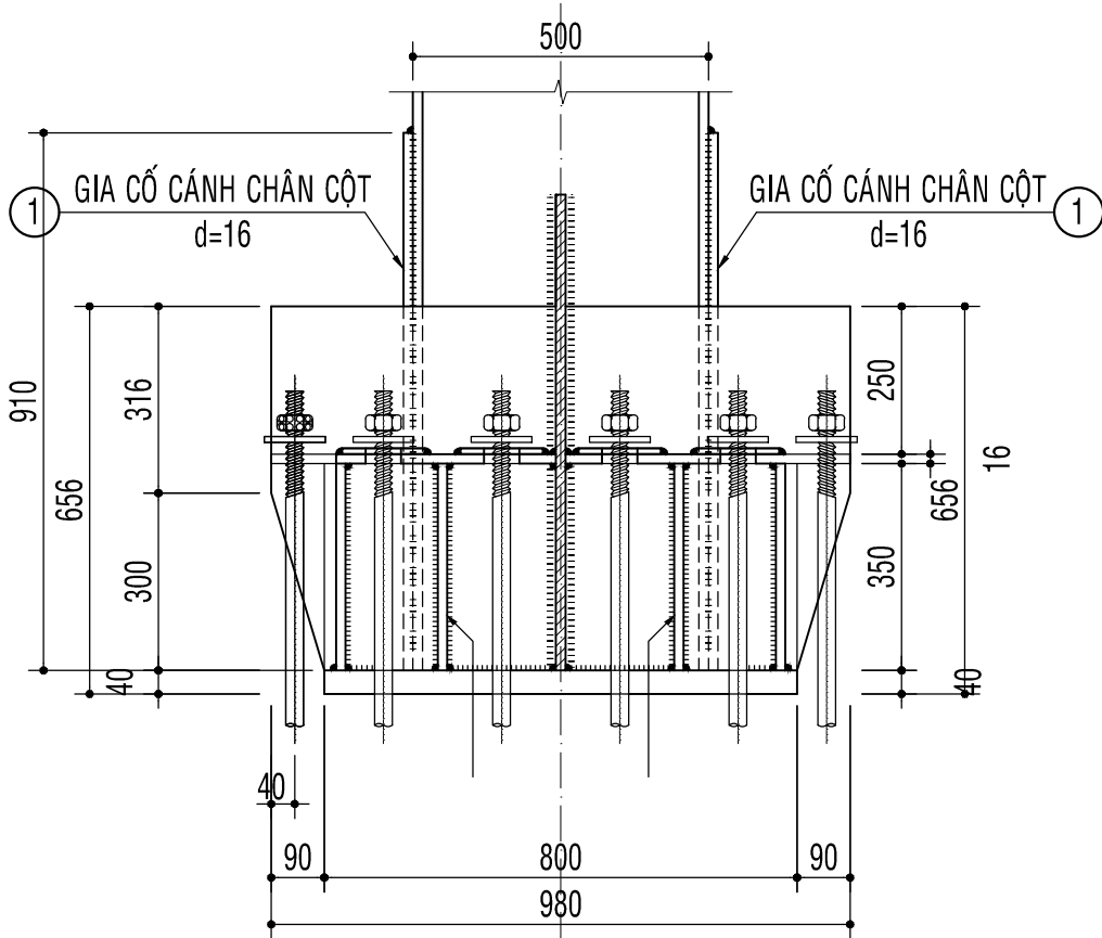
CẮT 3-3
