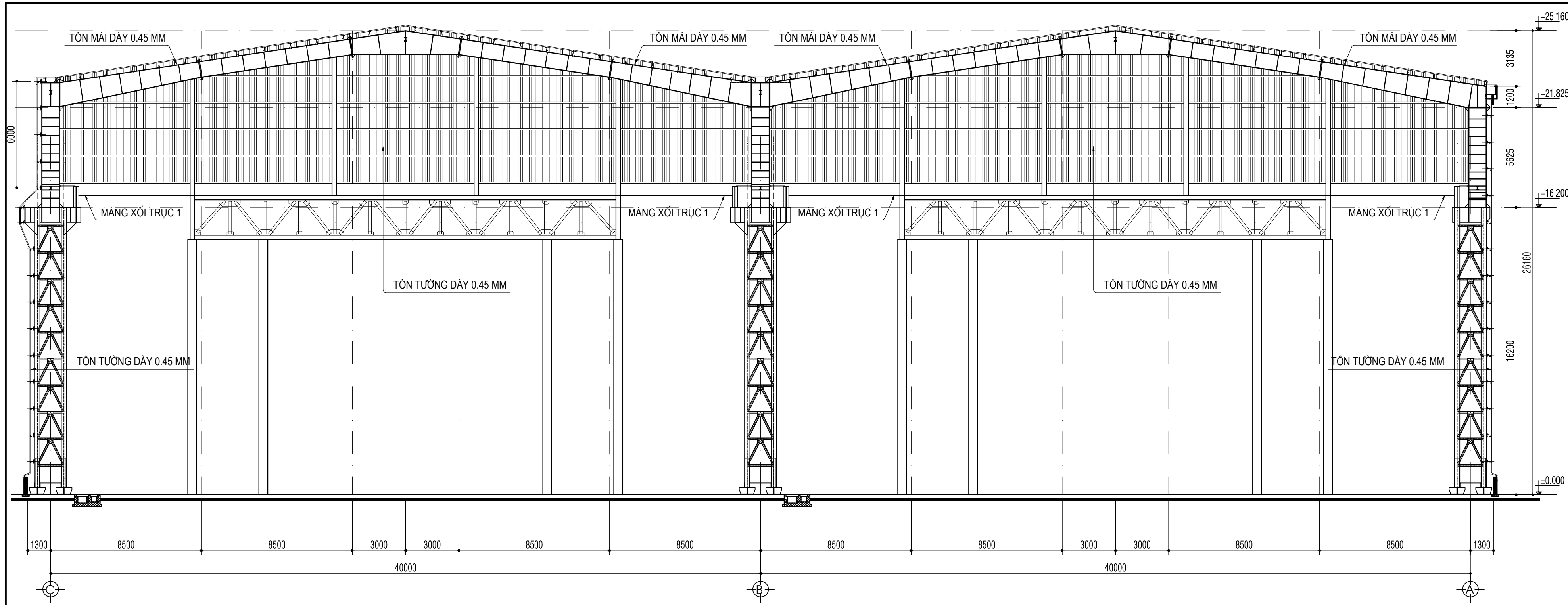
MẶT CẮT A-A - TL1/100
