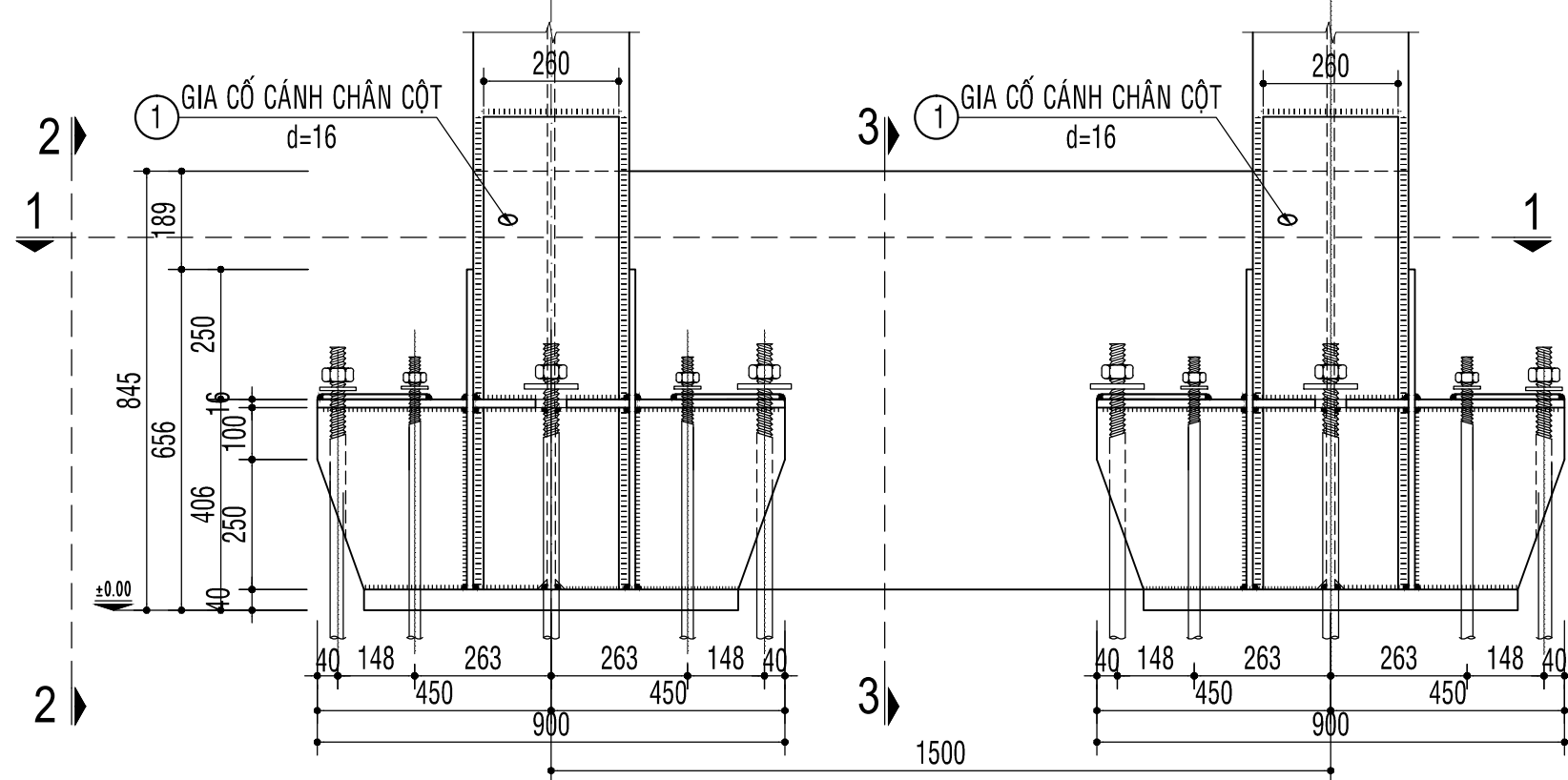
CHÂN CỘT
