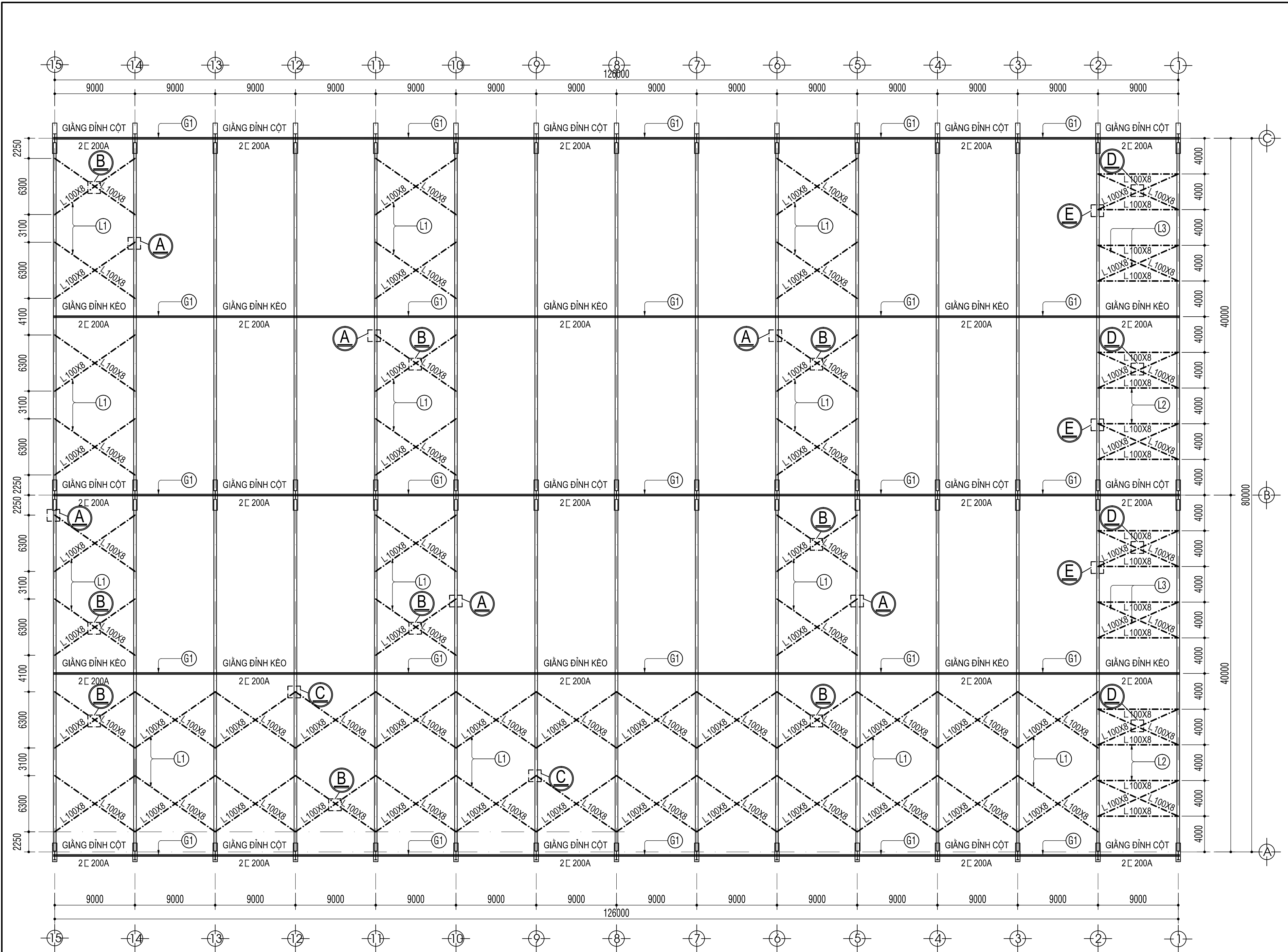
SƠ ĐỒ CẢI TẠO GIẢNG CÁNH TRÊN KÈO MÁI + GIẢNG ĐÌNH KÈO, ĐÌNH CỘT- TL 1/200
