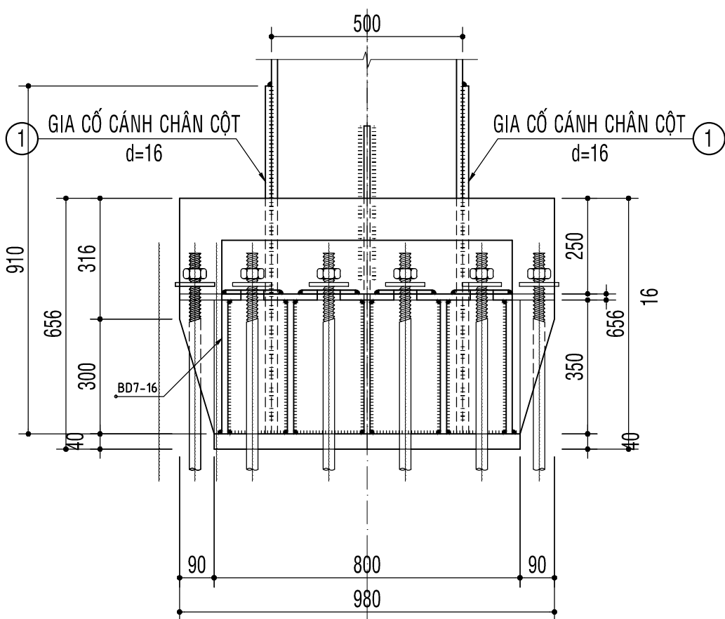
CẮT 2-2
