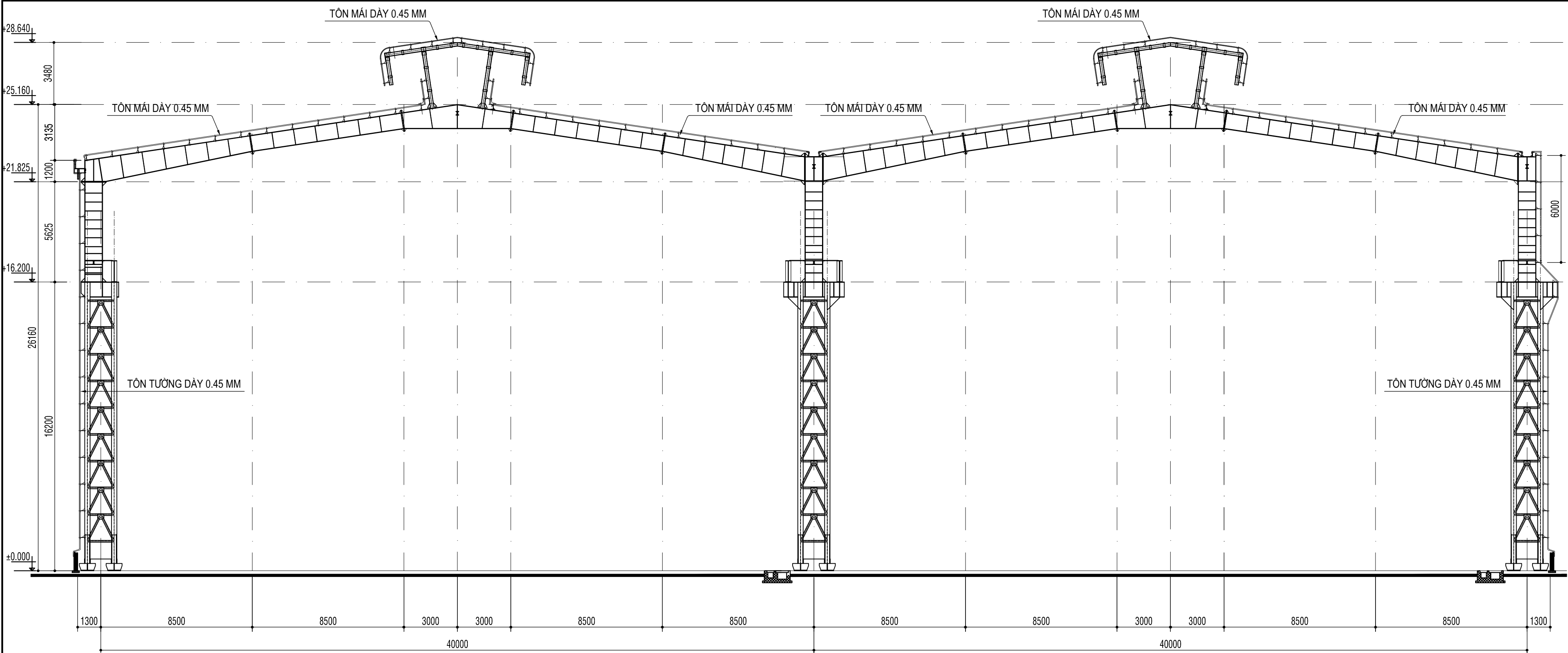
MẶT CẮT B-B - TL1/100
