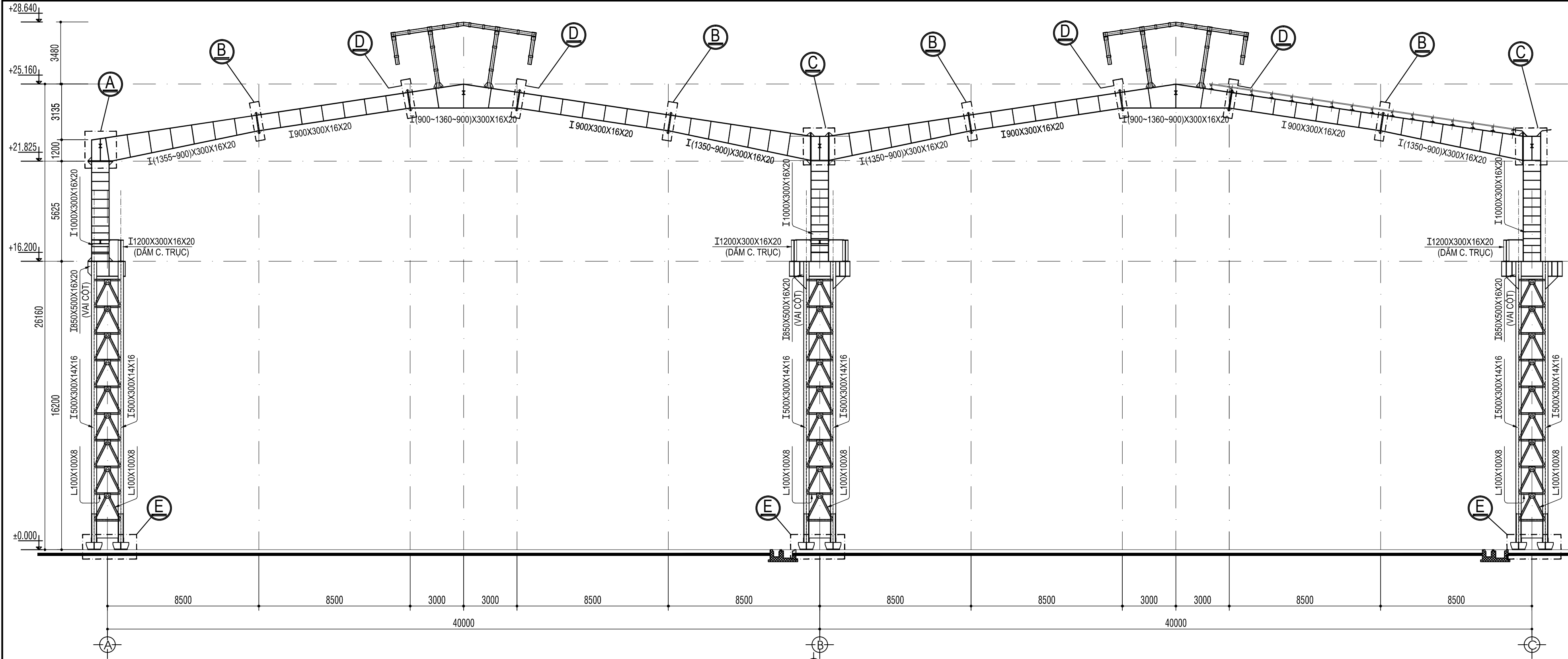
MẶT CẮT NGANG HIỆN TRẠNG- TL1/100
