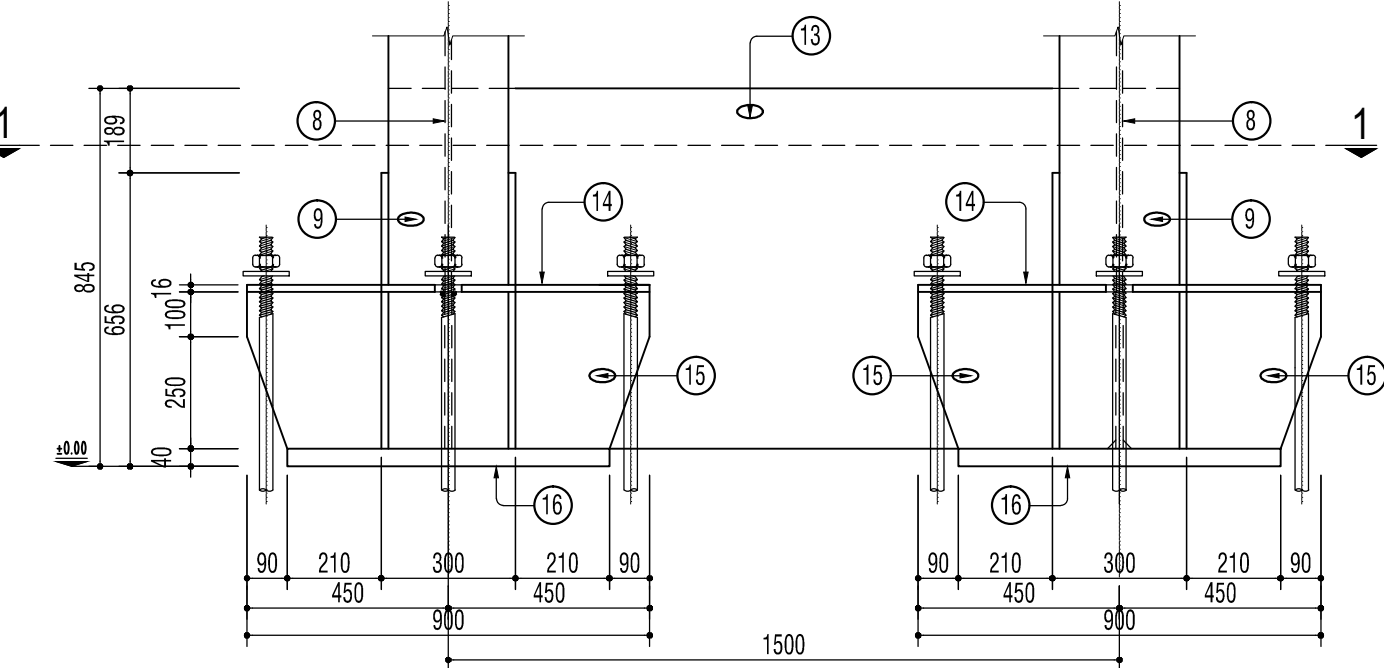
CHI TIẾT A3
