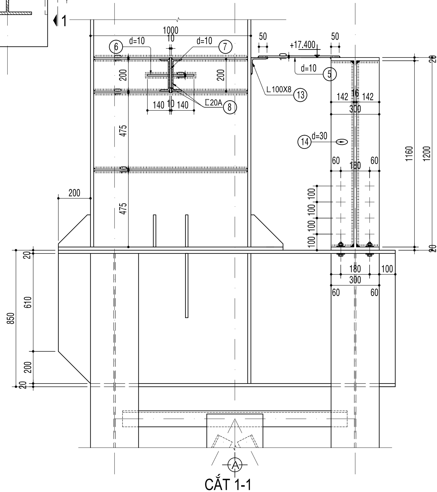
CHI TIẾT DẦM CẢN TRỤC, DẦM HẦM TRỤC A
