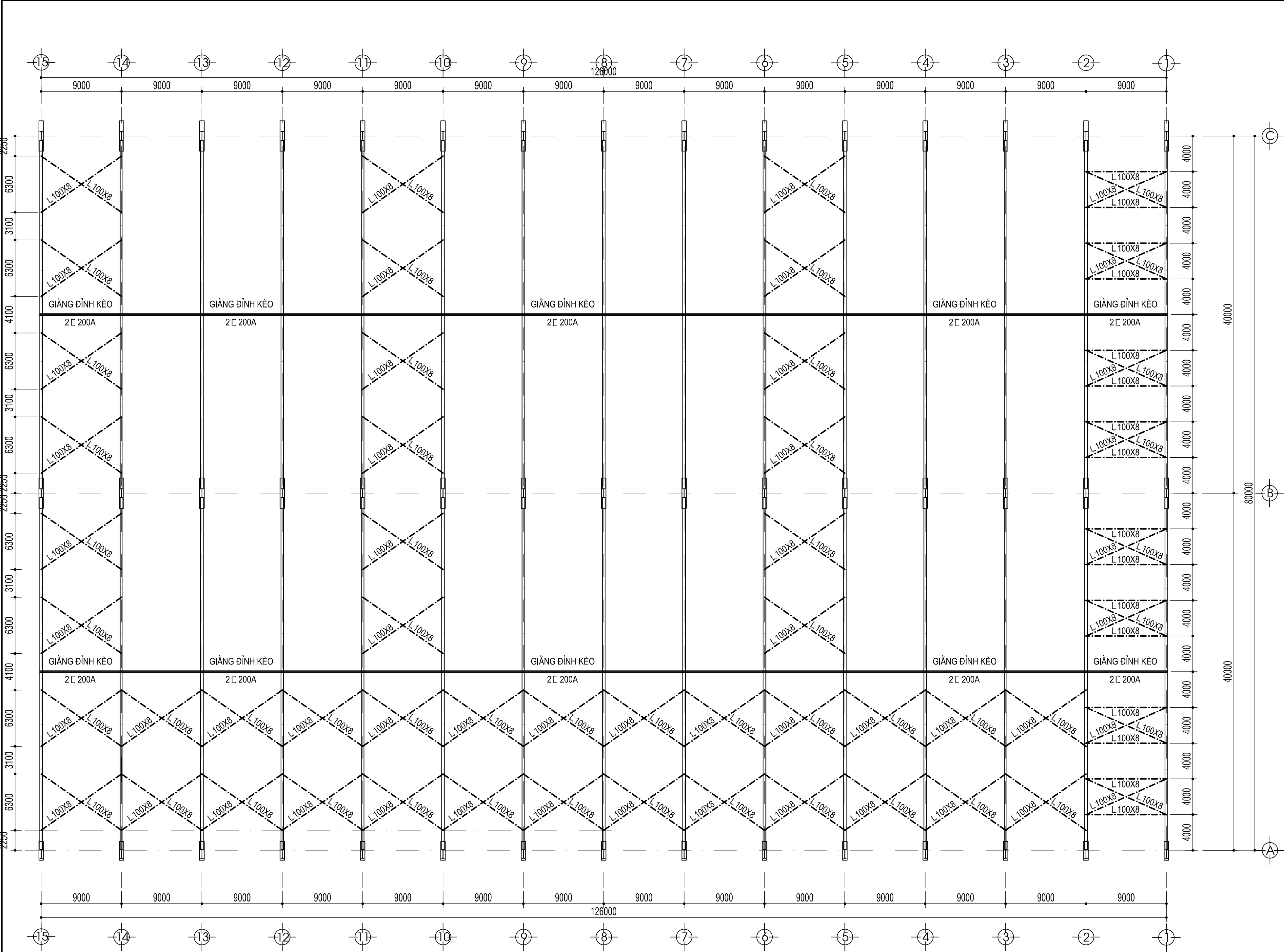
MẶT BẰNG HIỆN TRẠNG GIĂNG CÁNH TRÊN KÈO MÁI - TL 1/200
