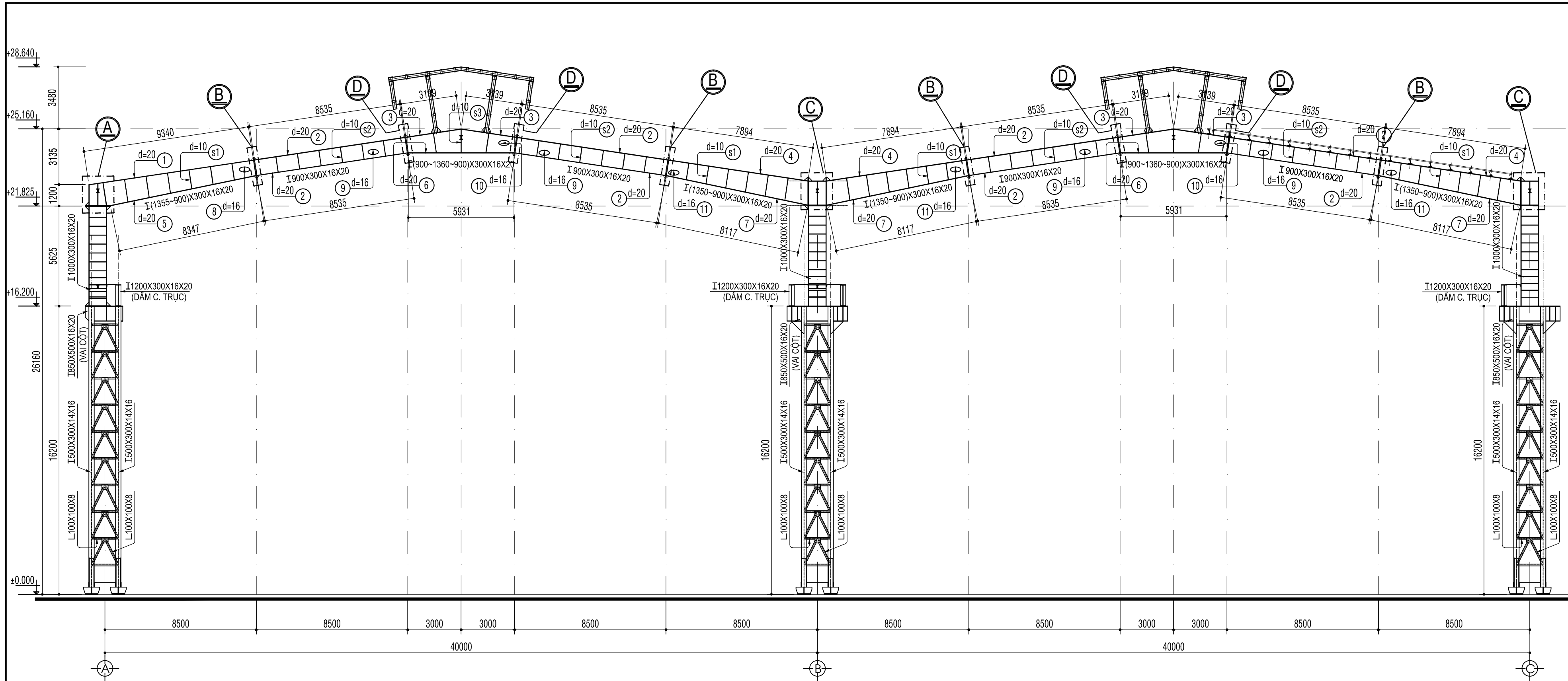
SƠ ĐỒ KHUNG GIỮ LẠI VỆ SINH ĐỂ CẢI TẠO
