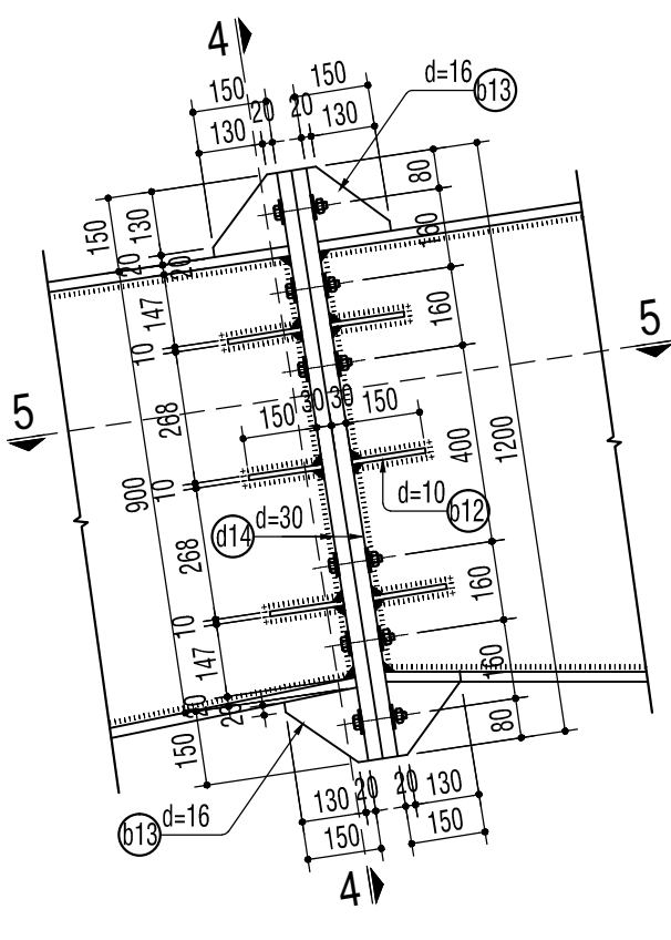
CHI TIẾT D BL: 12M30-8.8
