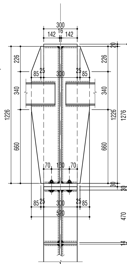
CẮT 2-2
