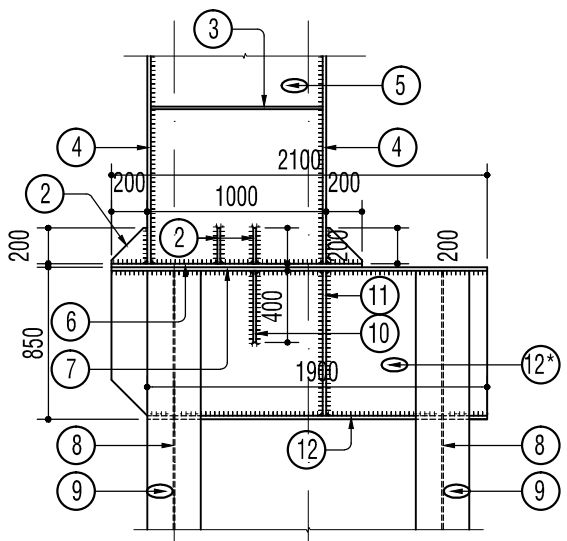
CHI TIẾT A2 12 BL M24(8.8)
