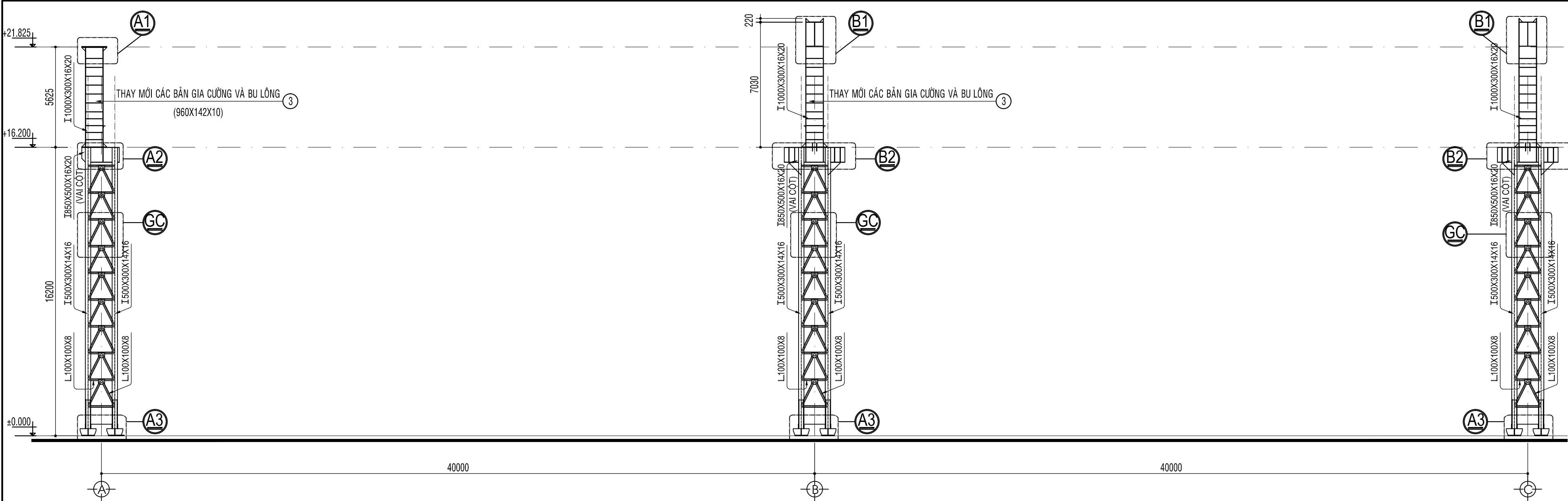
MẶT ĐỨNG CỘT GIỮ LẠI VỆ SINH ĐỂ CẢI TẠO TRỤC A-C
