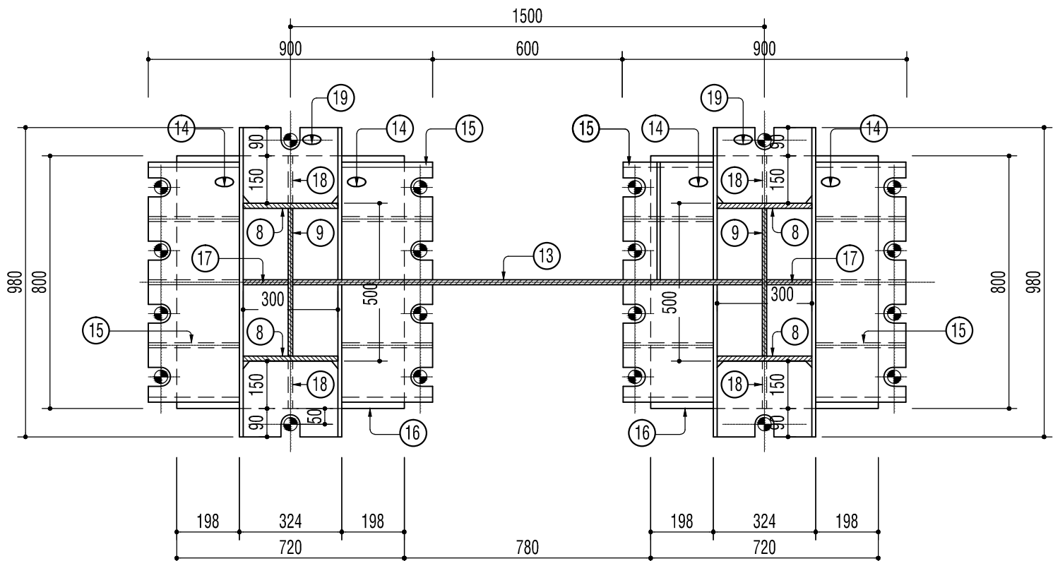
CẮT 1-1
