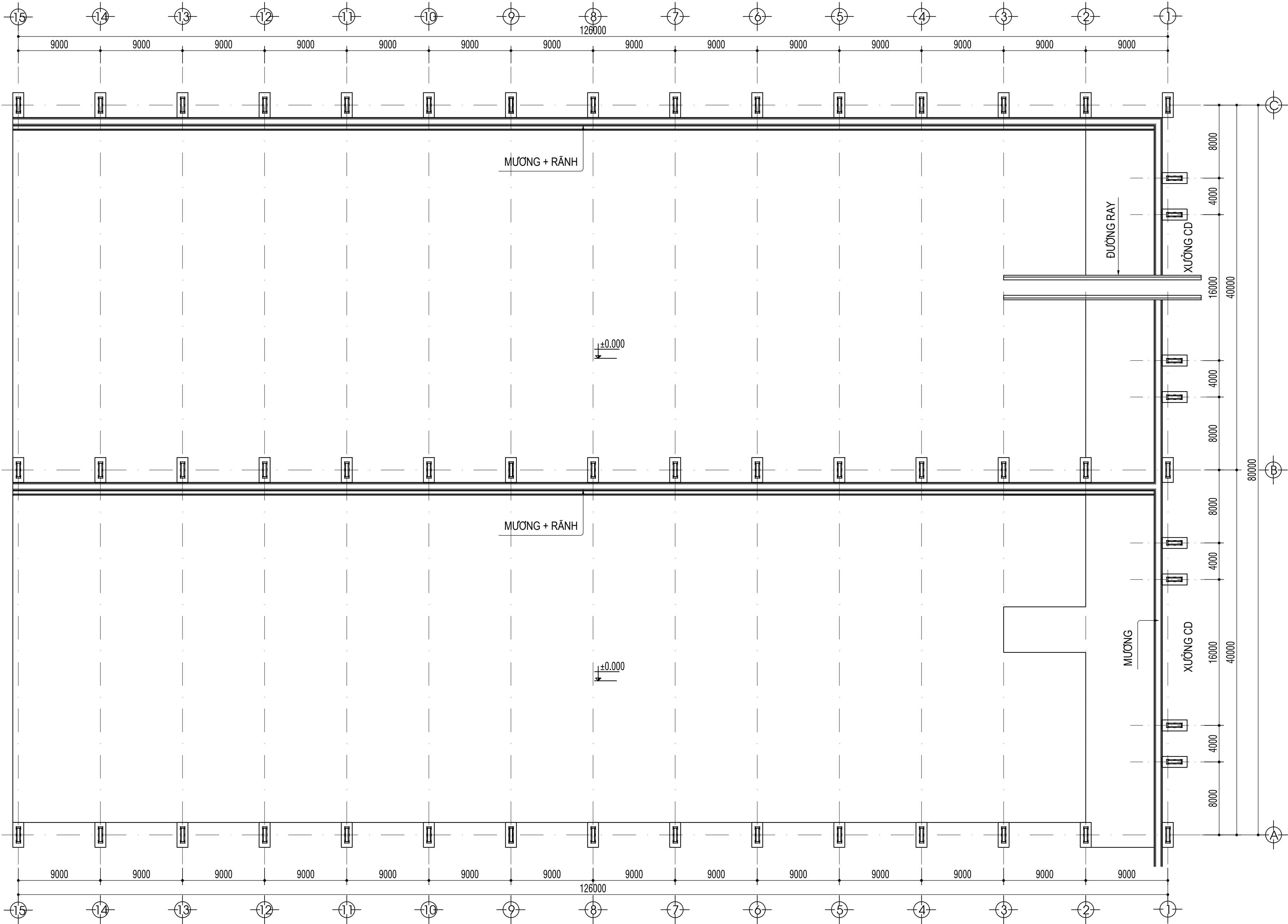
MẶT BẰNG HIỆN TRẠNG COTE ±0.000 - TL1/200
