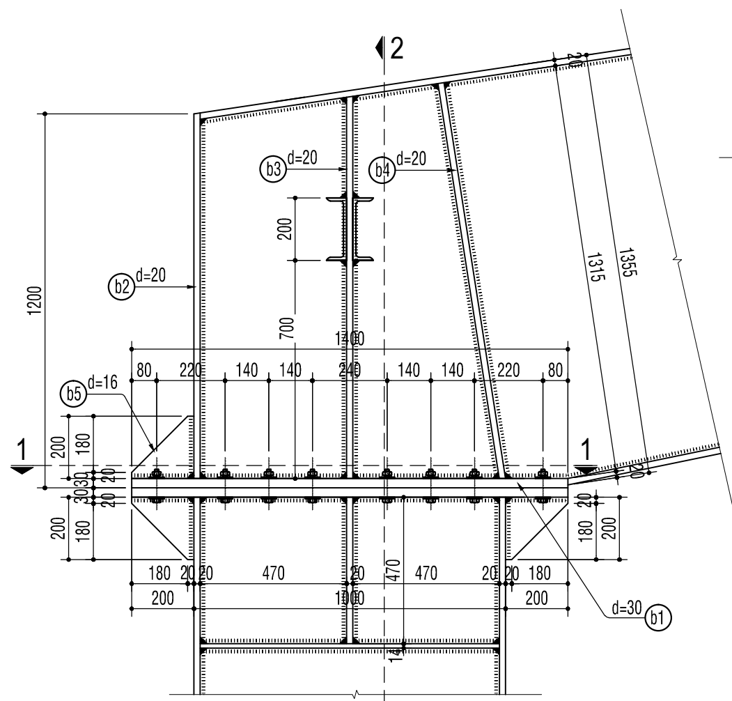
CHI TIẾT A
