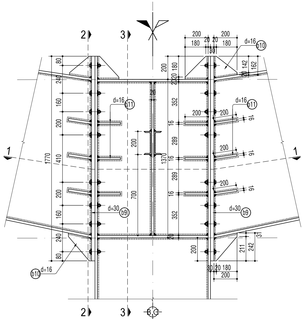
CHI TIẾT C BL: 32M30-8.8
