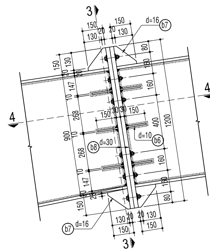
CHI TIẾT B
