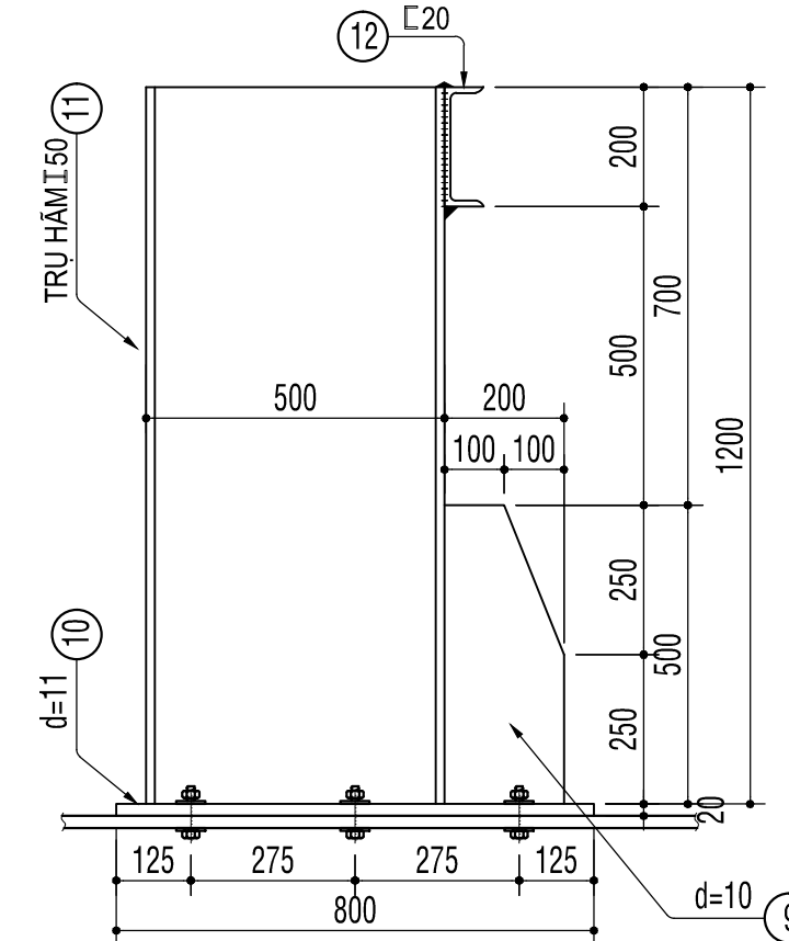
CẮT 5-5
