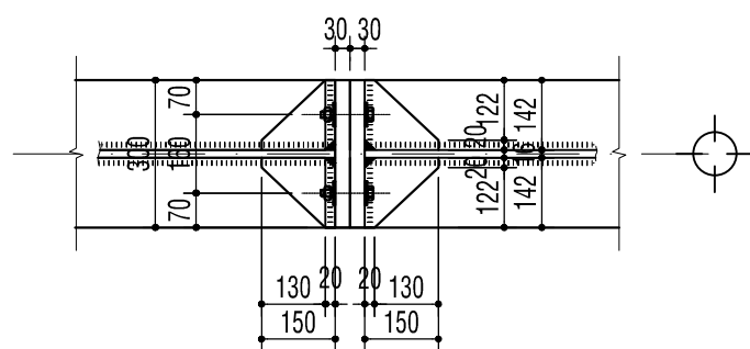
CẮT 4-4
