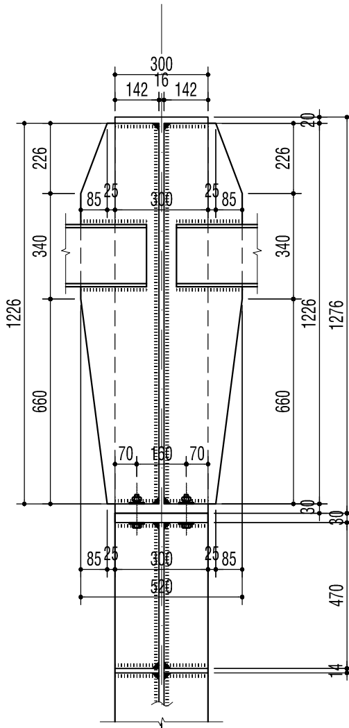
CẮT 2-2
