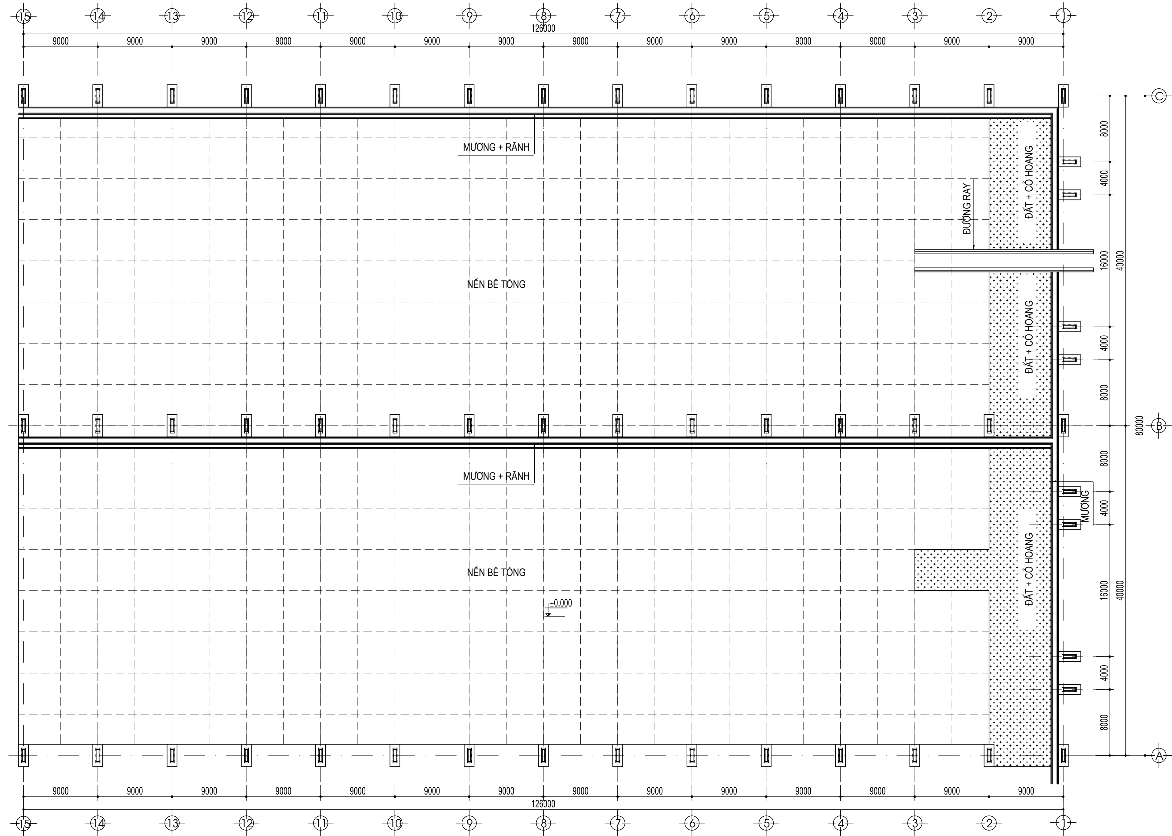
MẶT BẰNG NỀN HIỆN TRẠNG COTE ±0.000 - TL1/200
