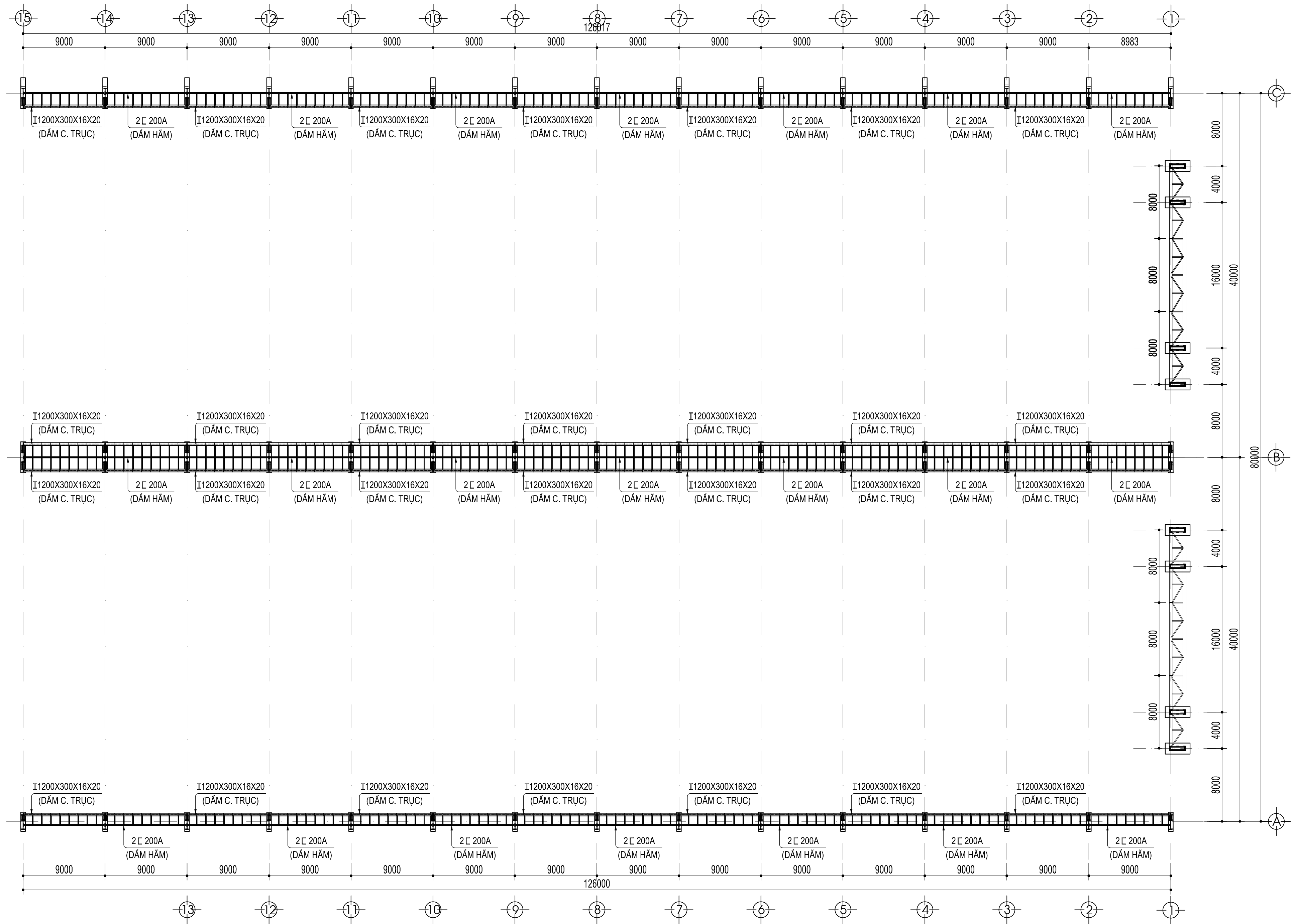
DẦM CẦU TRỤC GIỮ LẠI VỆ SINH ĐỂ CẢI TẠO
