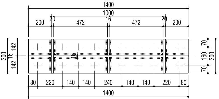
CẮT 1-1
