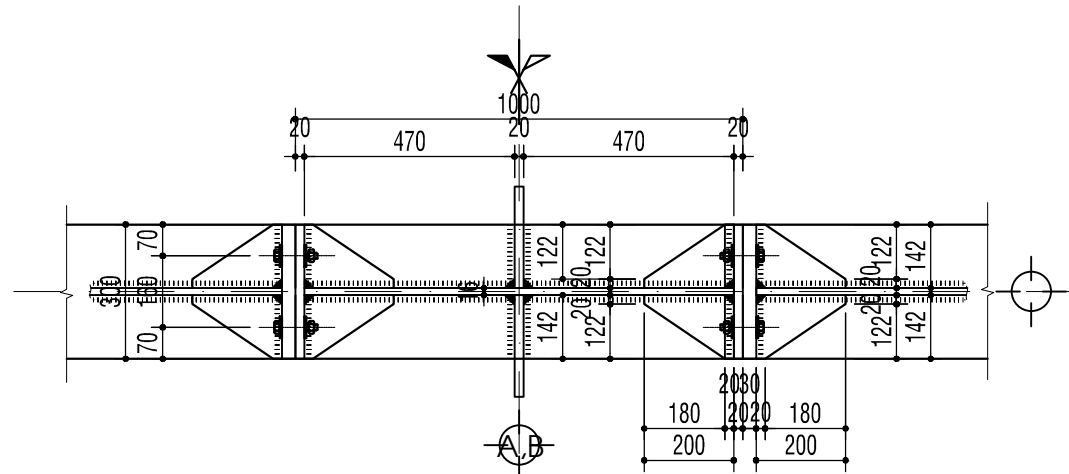
CẮT 1-1
