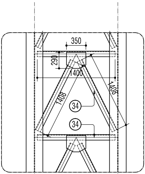
CHI TIẾT GC
