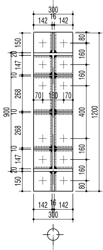
CẮT 4-4
