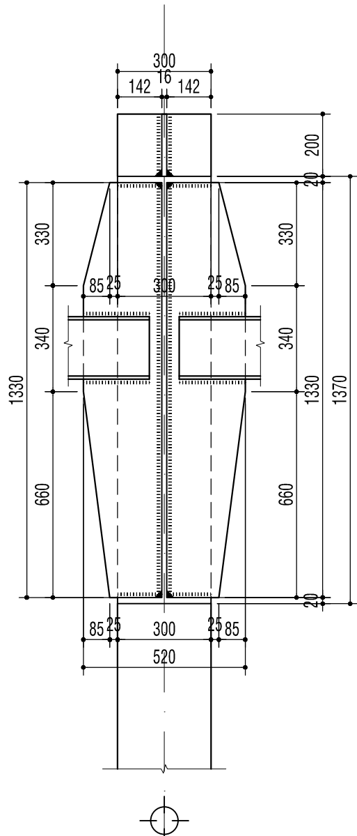
CẮT 3-3
