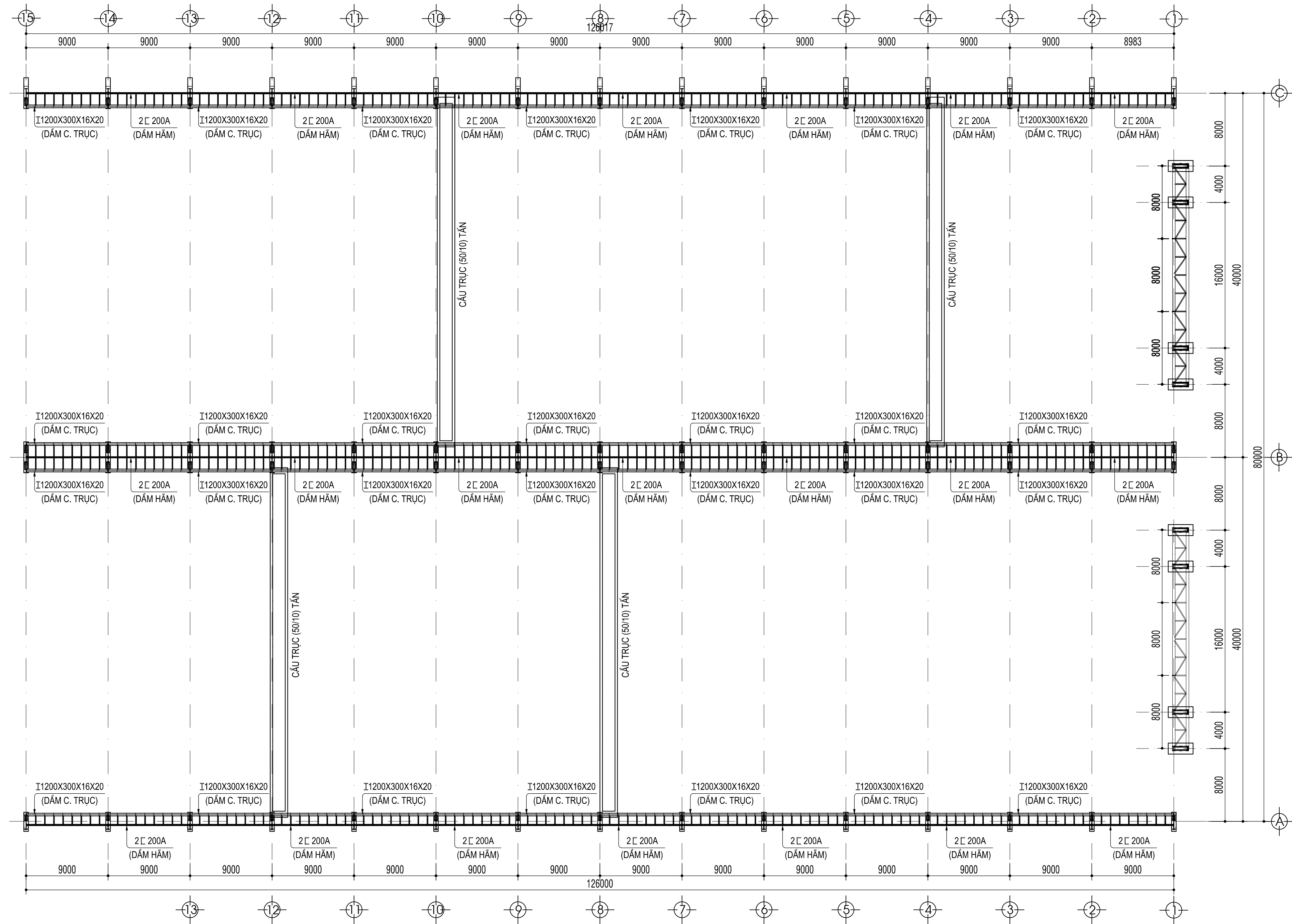
MẶT BẰNG HIỆN TRẠNG COTE + 18.000 - TL1/200
