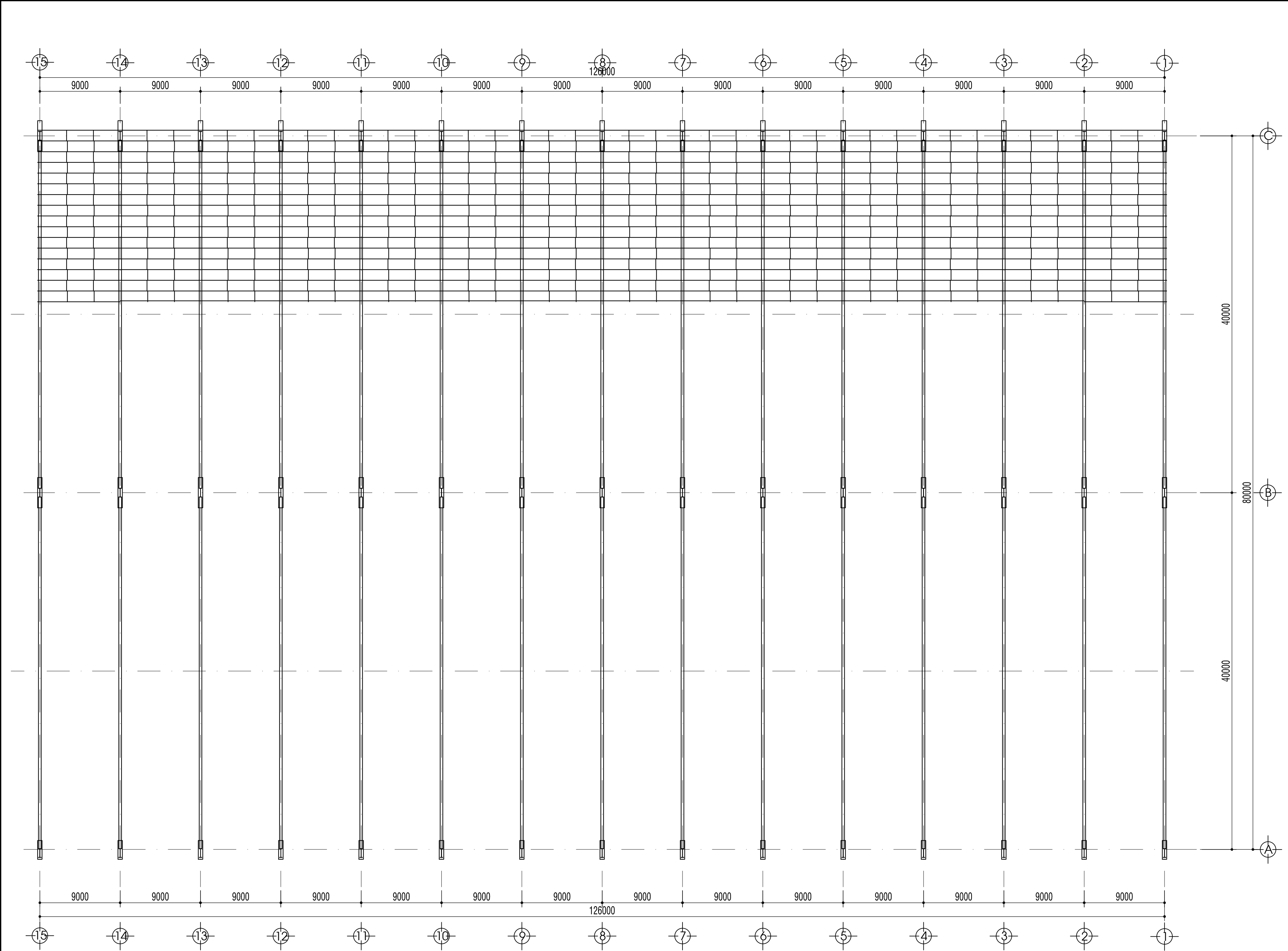
MẶT BẰNG HIỆN TRẠNG XÀ GỖ MÁI - TL1/200
