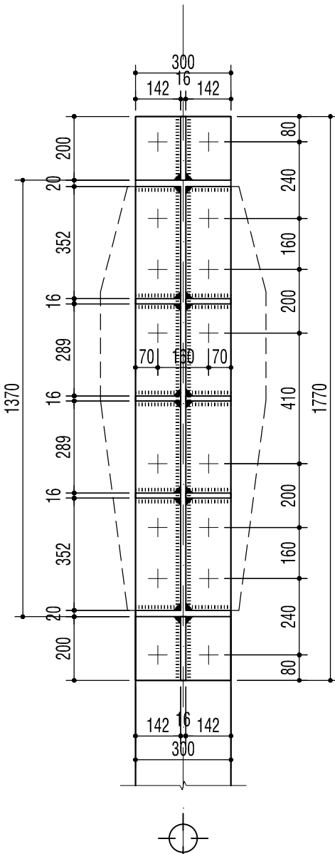
CẮT 2-2
