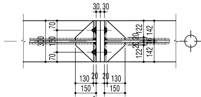
CẮT 5-5
