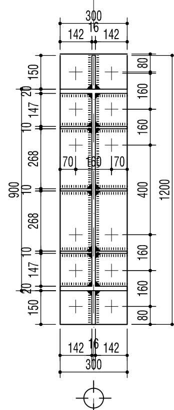
CẮT 3-3
