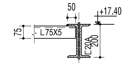
CẮT 3-3
