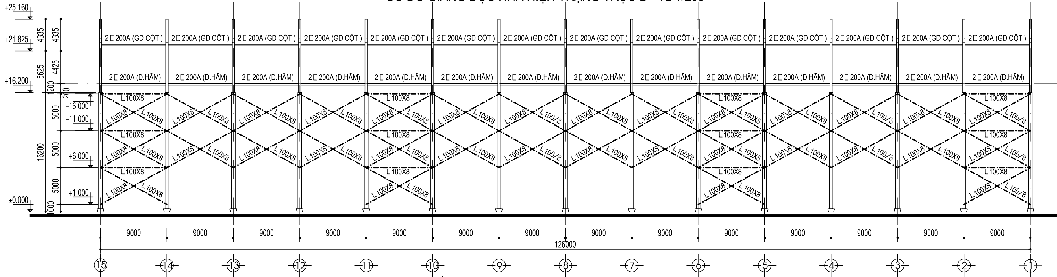
SƠ ĐỒ GIẺNG DẠC NHÀ HIỆN TRẠNG TRỤC C - TL 1/200
