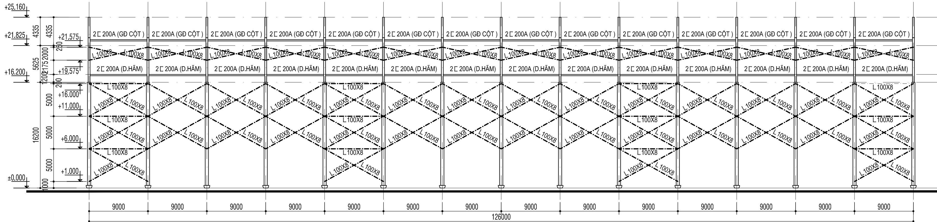
SƠ ĐỒ GIẺNG DẠC NHÀ HIỆN TRẠNG TRỤC A - TL 1/200
