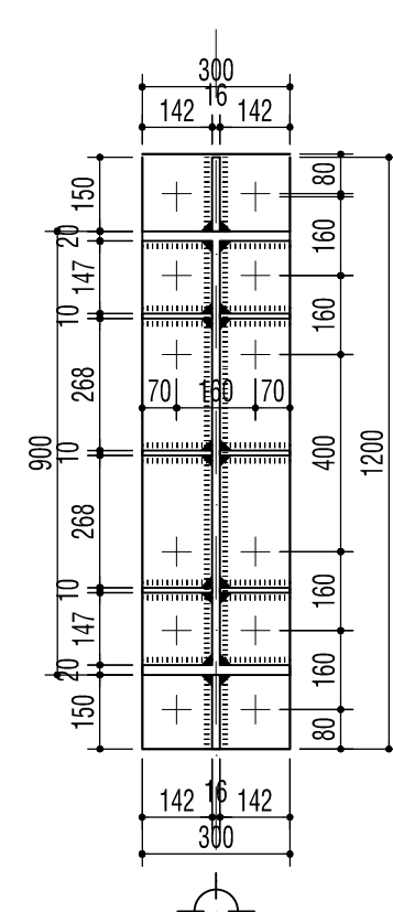
CẮT 3-3
