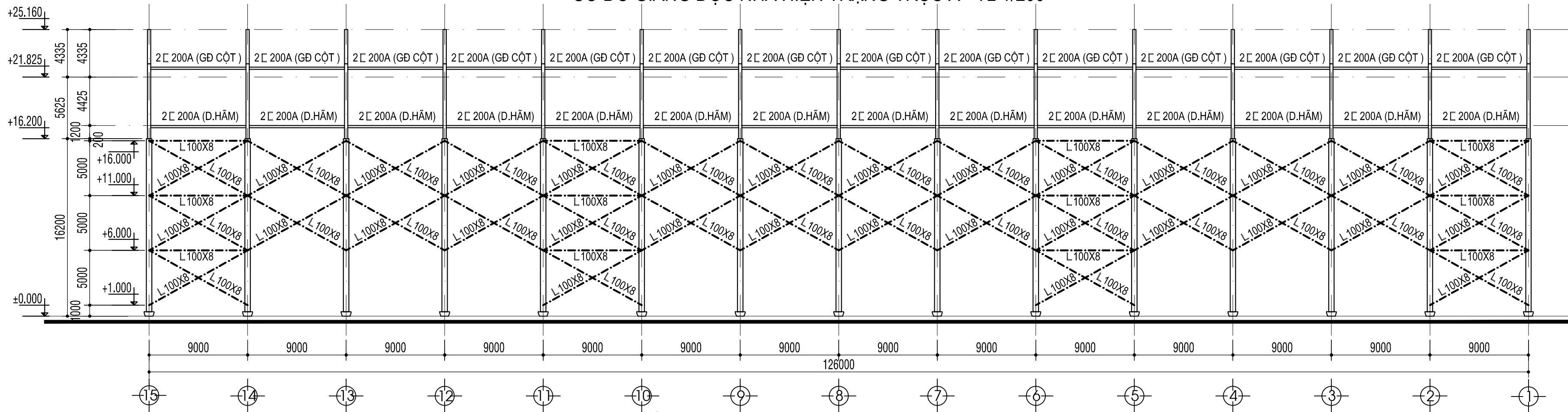
SƠ ĐỒ GIẺNG DẠC NHÀ HIỆN TRẠNG TRỤC B - TL 1/200
