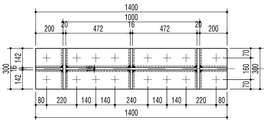
CẮT 1-1
