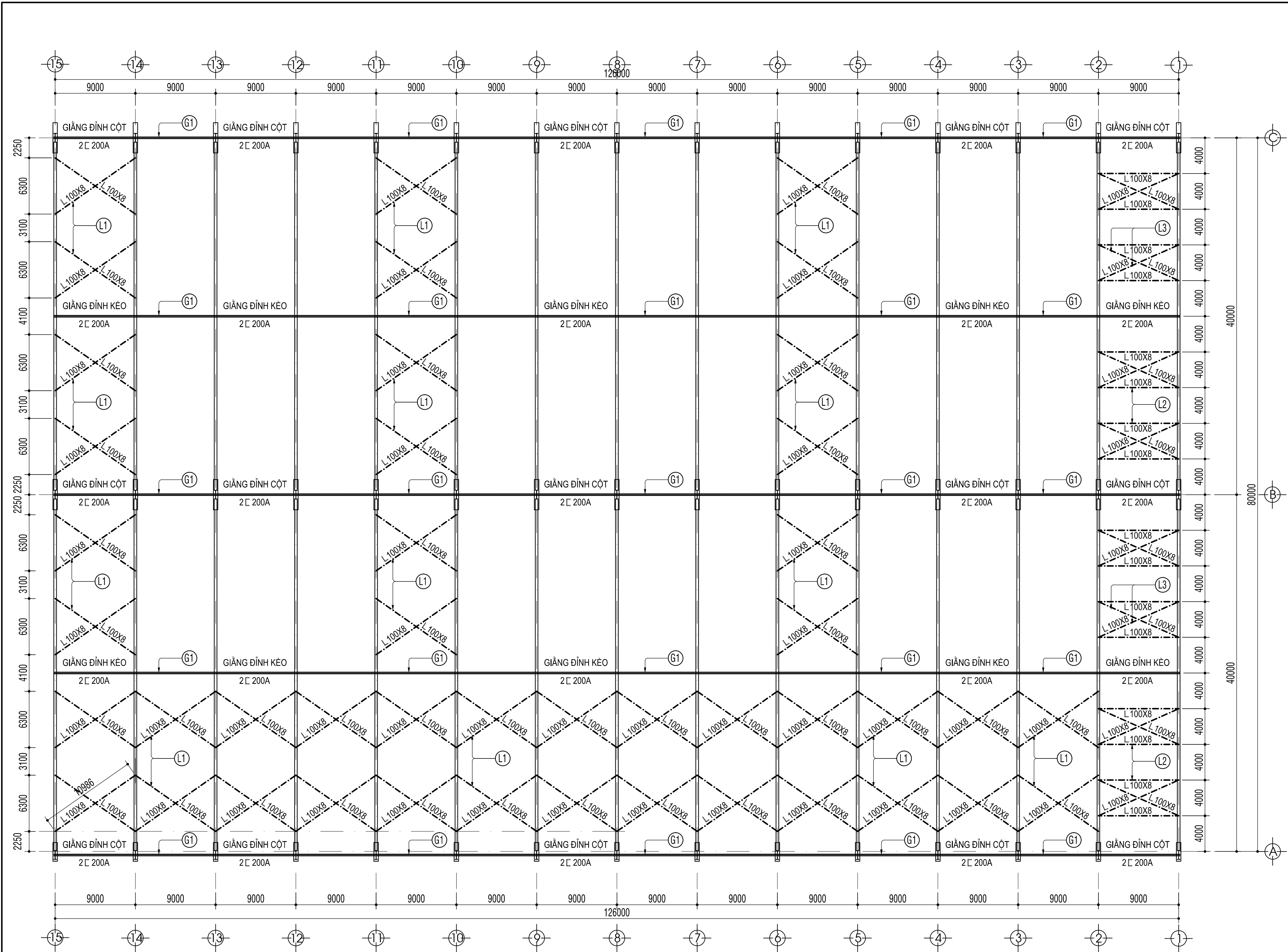
THẢO DỒ GIẺNG CÁCH TRÊN KÈO MÁI + GIẺNG ĐỈNH KÈO, ĐỈNH CỘT - TL 1/200
